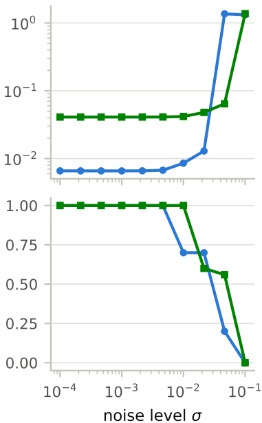
Lorenz
