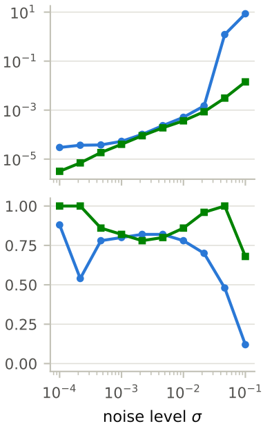
Lotka-Volterra
