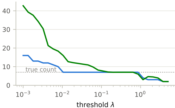
Lorenz
