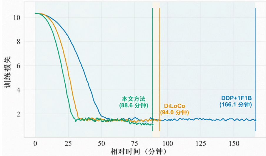
图 5.6 训练 loss 随墙钟时间变化：POLAR-SGD 更快进入低 loss 区间
