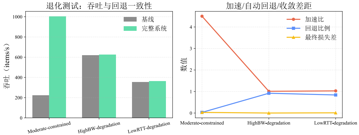
图 6.5 高带宽/低 RTT 退化测试下的自动回退与一致性验证
