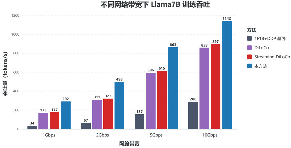
图 6.3 不同跨域带宽下 LLaMA-7B 训练吞吐的横向方法对比
