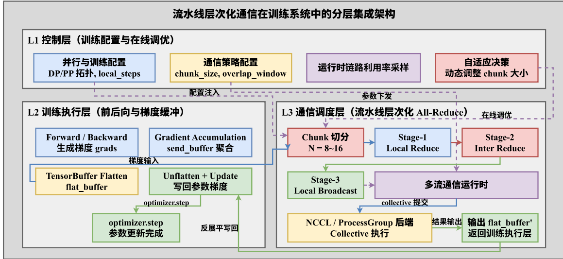
图 4.4 流水线调度器在训练流程中的集成架构
