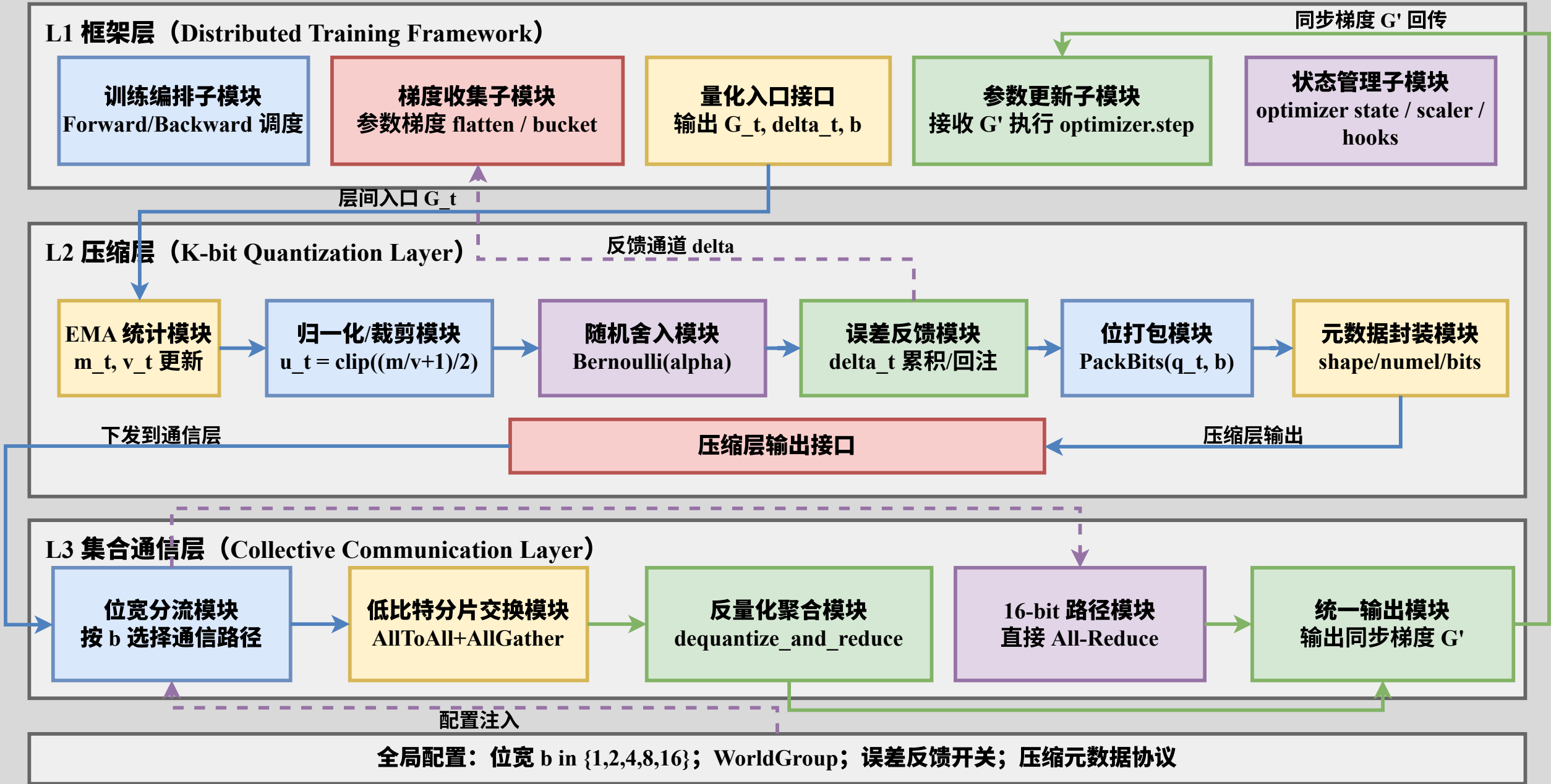
统一 k-bit 随机舍入量化细粒度分层架构图 (Framework → Compression → Collective)
