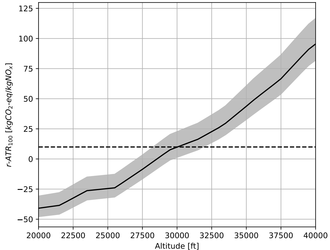
NOx
