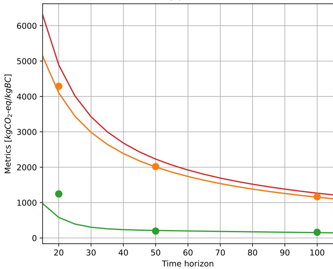
(e) Soot
