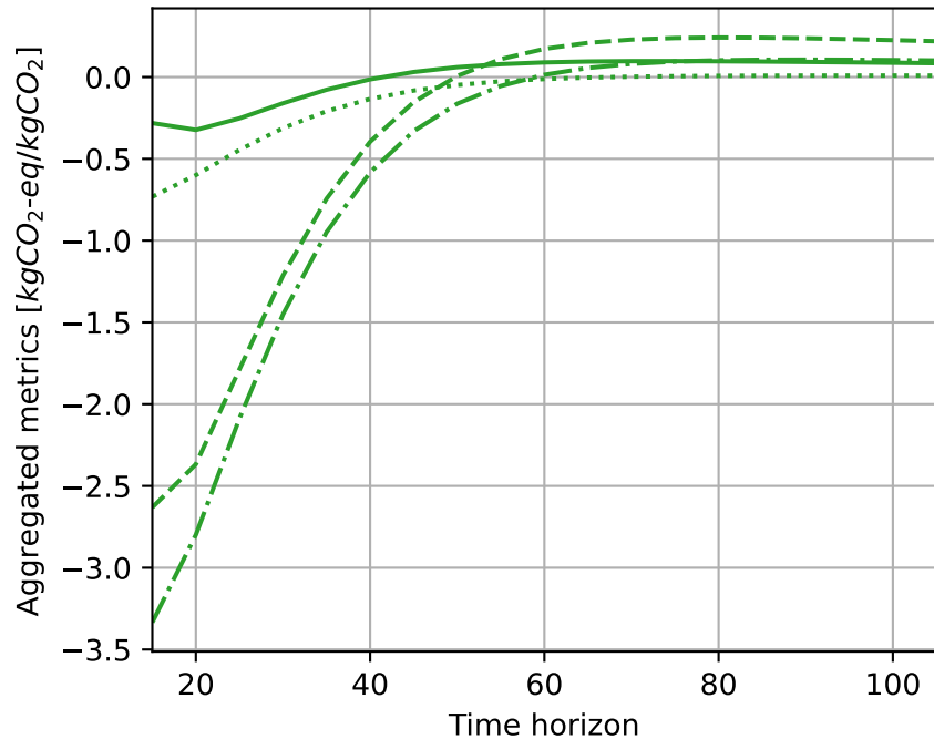
(b) GTP
