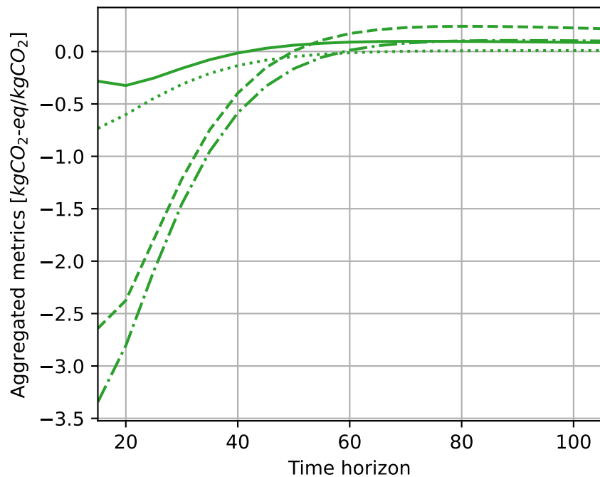
(b) GTP
