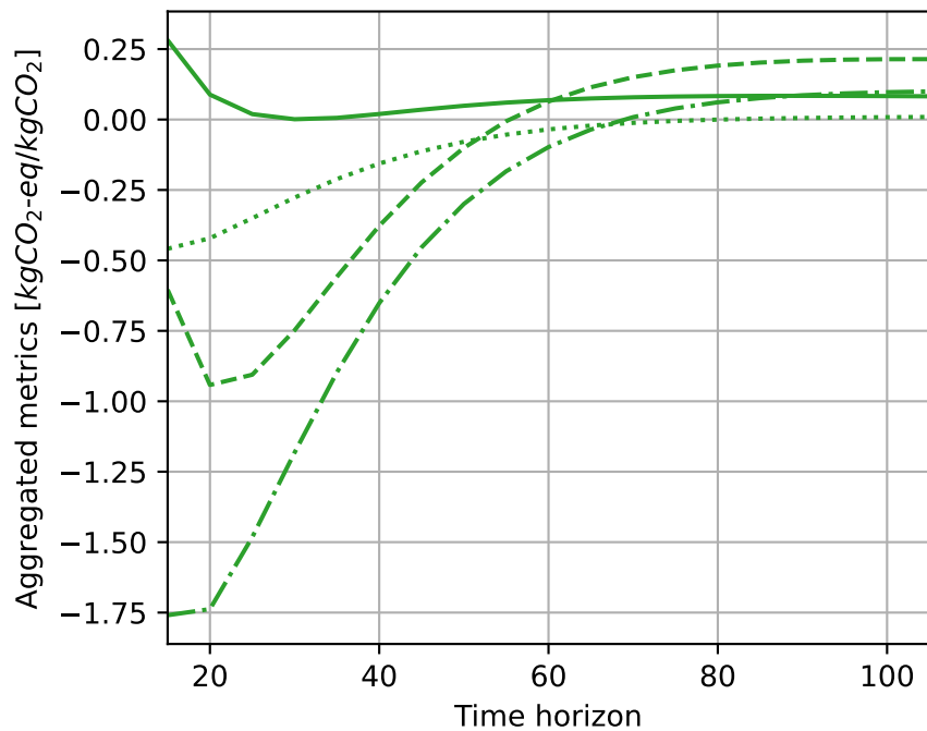
(b) GTP
