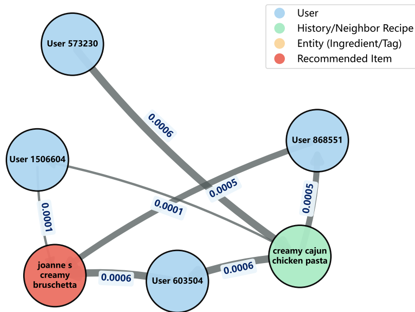
Figure 4.3: 案例 B：協同過濾路徑示意圖 (User 573230)
