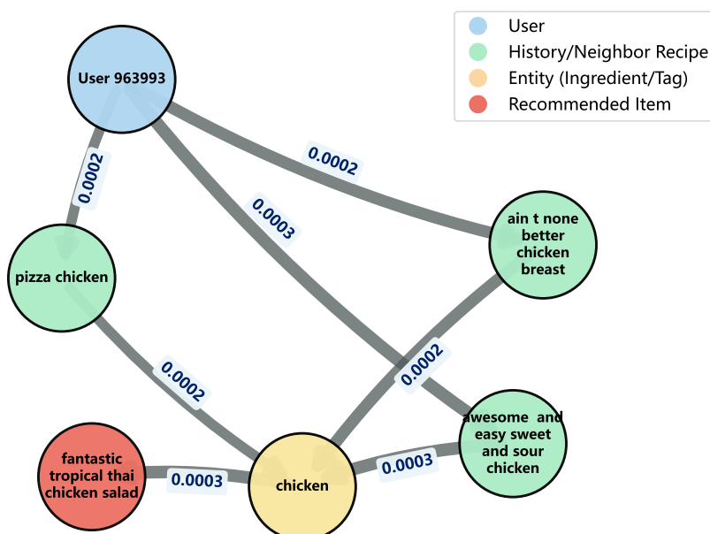
Figure 4.4: 案例 C : KG 語意路徑示意圖 (User 963993)
