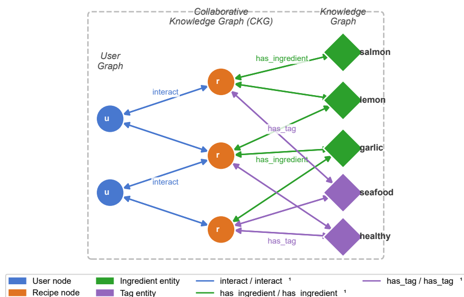
Figure 3.2: 協同知識圖 (CKG) 架構示意：整合使用者-食譜互動圖與食譜知識圖，包含互動、食材與標籤三類關係邊。
