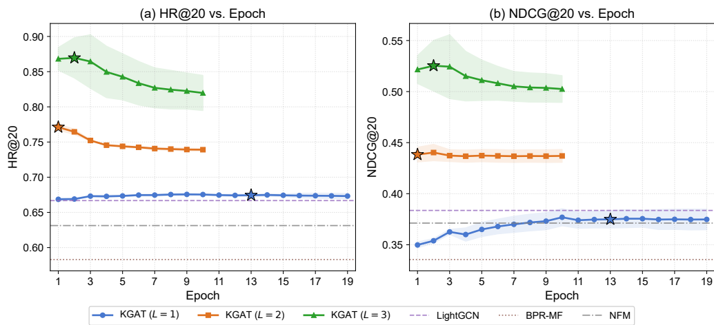
Figure 4.1: 不同傳播深度 KGAT 模型的訓練過程比較，含三條 Baseline 水平基線。
