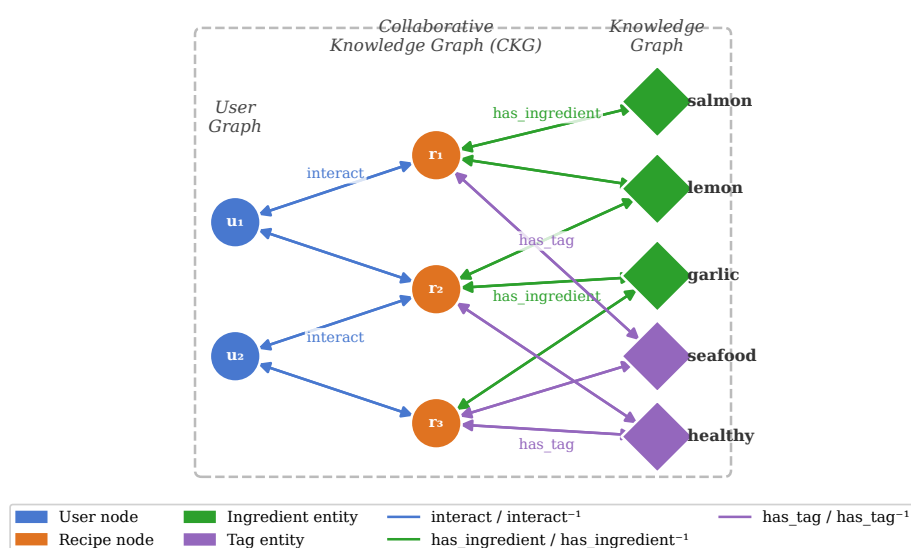
Figure 3.2: 協同知識圖 (CKG) 架構示意：整合使用者-食譜互動圖與食譜知識圖，包含互動、食材與標籤三類關係邊。
