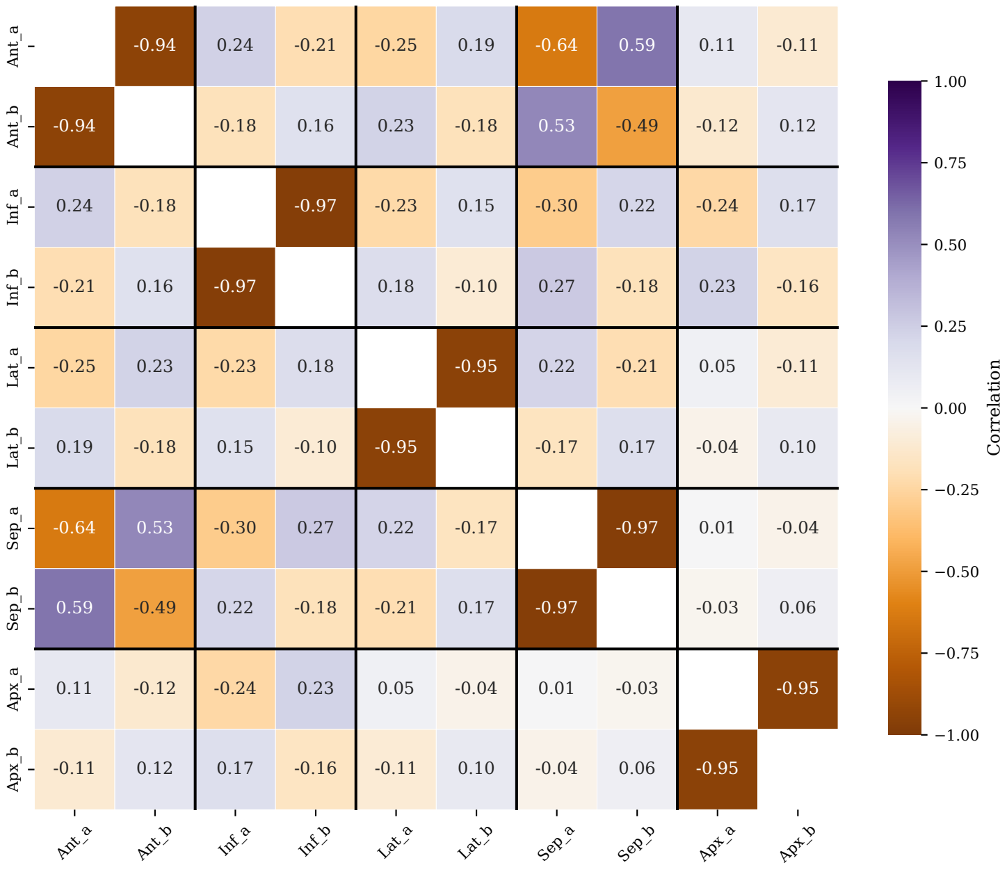
Full Parameter Correlation — MI Mild ( \mu=1.5 )
