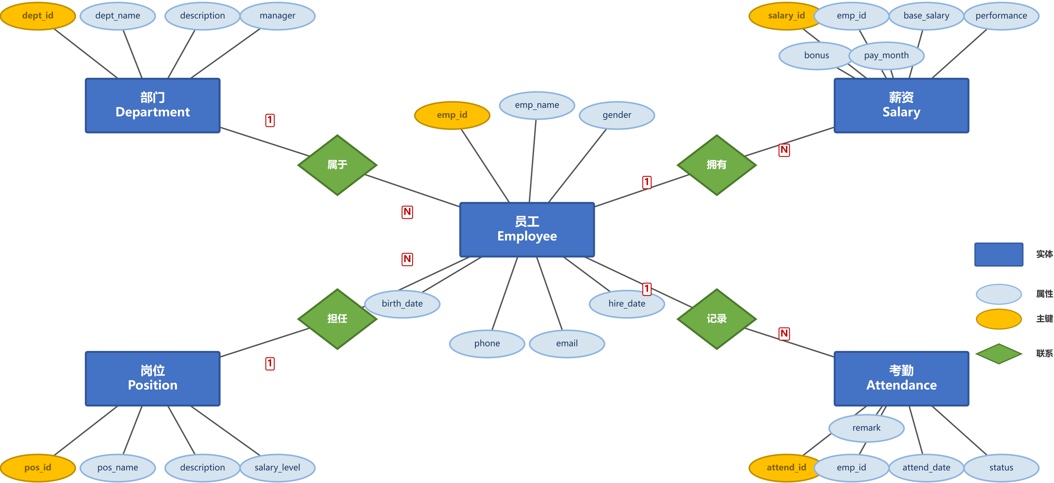
企业员工管理系统 E-R 图
