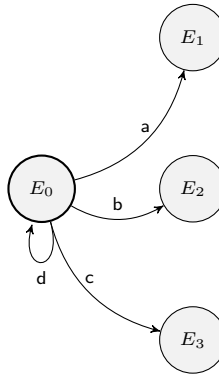
FIGURE 6 – Un noeud d'un automate ...
