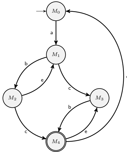
FIGURE 8 – Un automate accepteur
