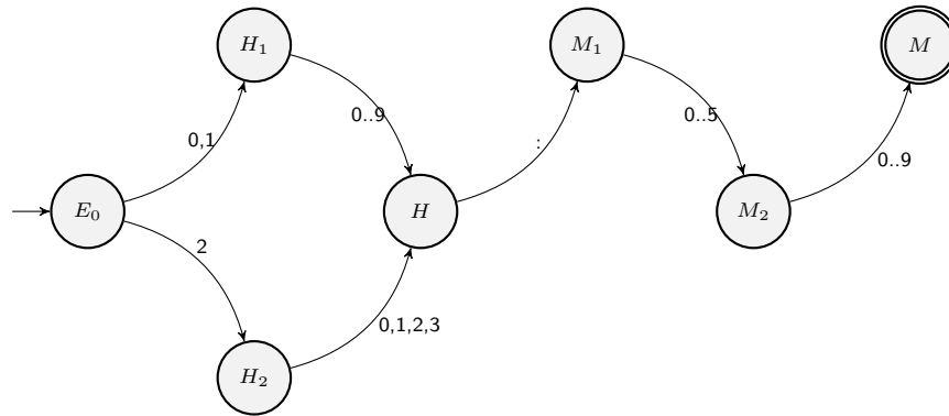
FIGURE 5 – Un automate accepteur
