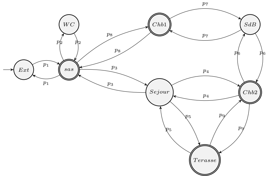
FIGURE 7 – Automate A_m du visiteur
