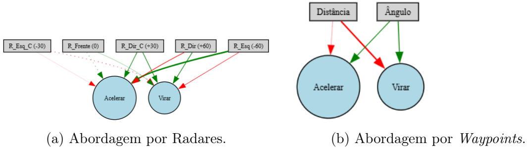
Figure 2: Topologias das redes neuronais dos controladores vencedores obtidos através do algoritmo NEAT.
