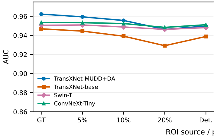
(a) Absolute AUC
