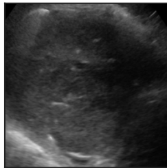
AUL
