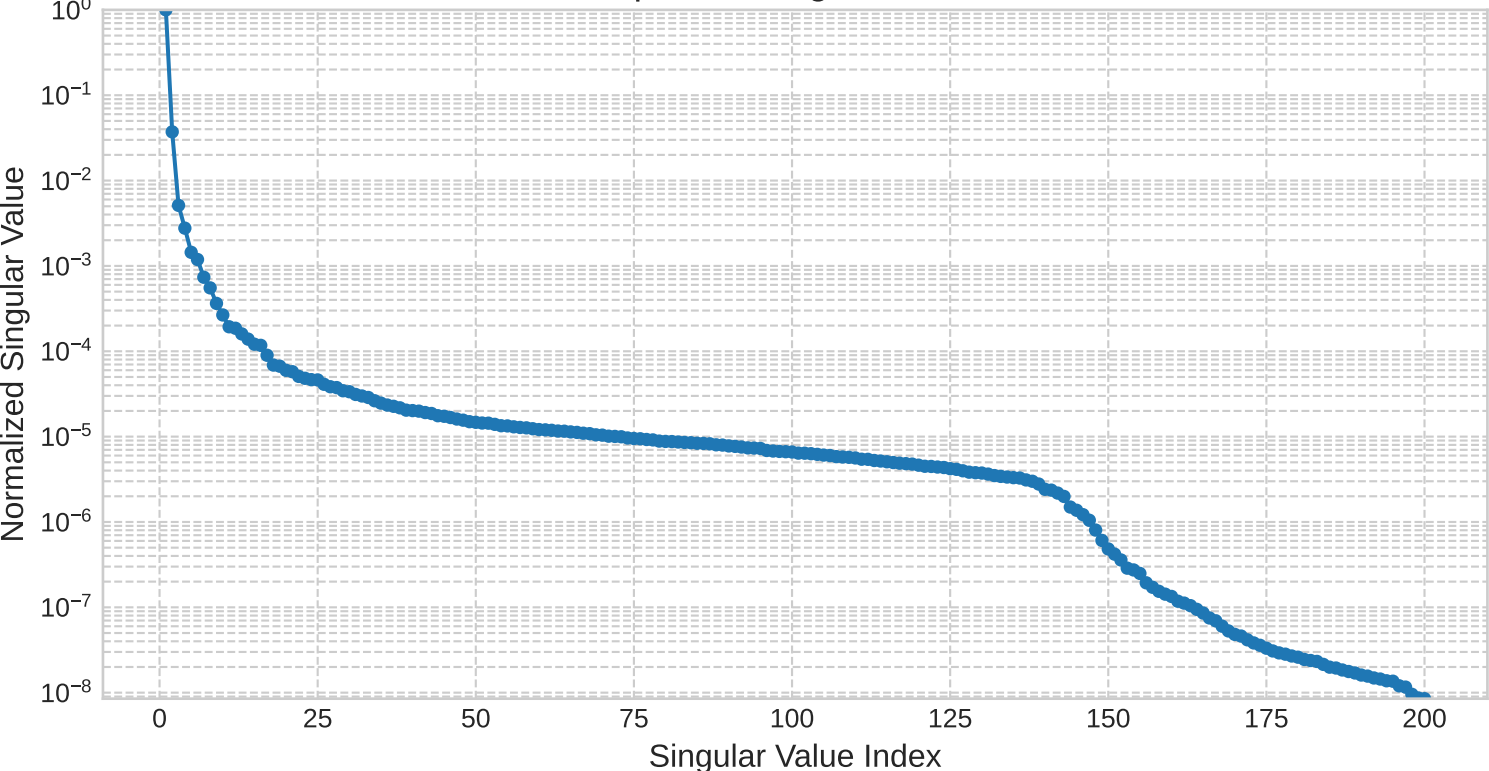
Amplitude Singular Values
