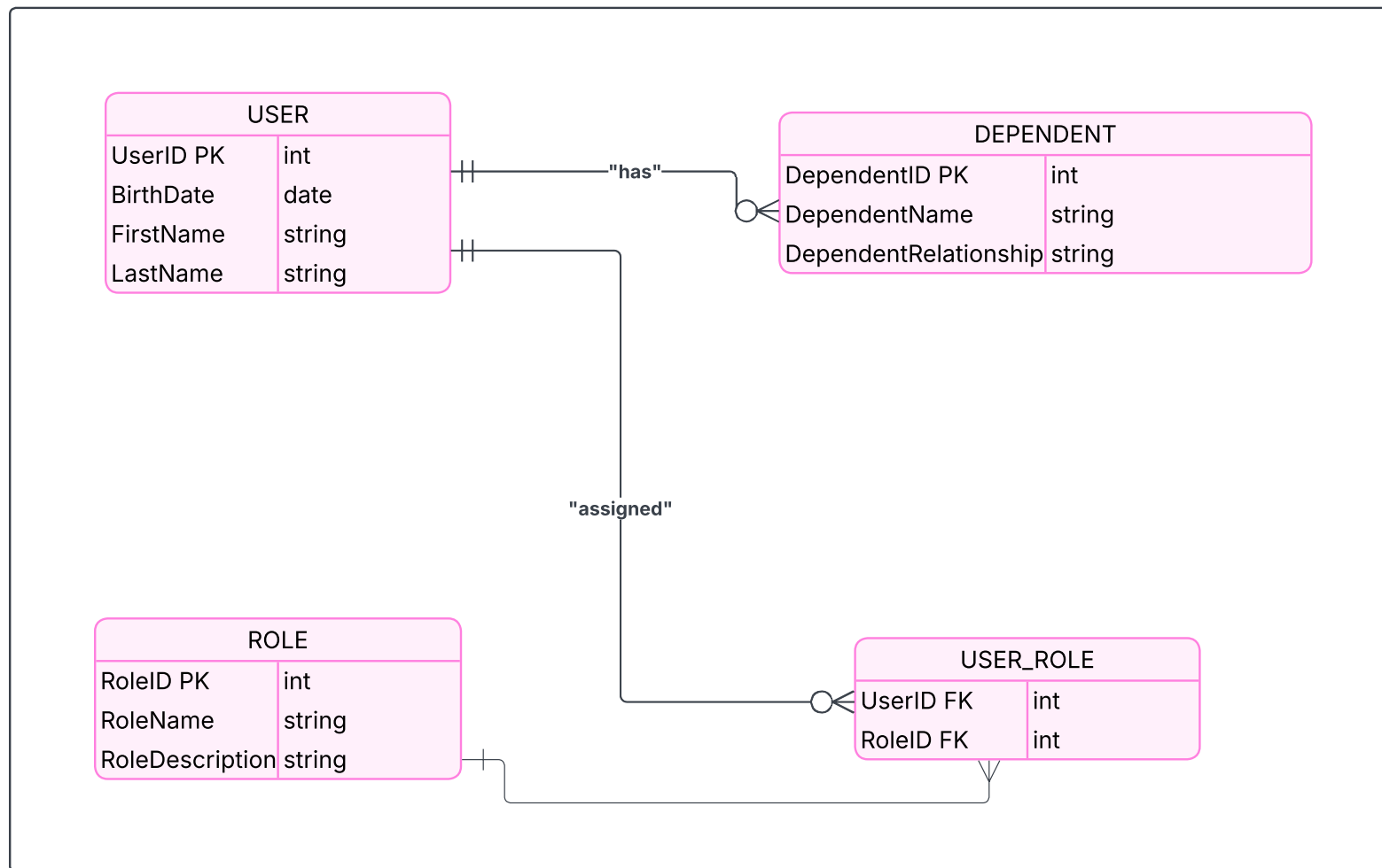
Entity-Relationship Diagram (ERD)
