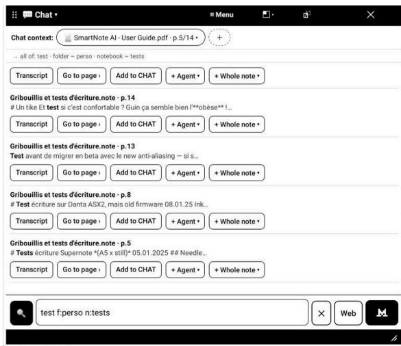
Fig. 5.3, Search mode.
