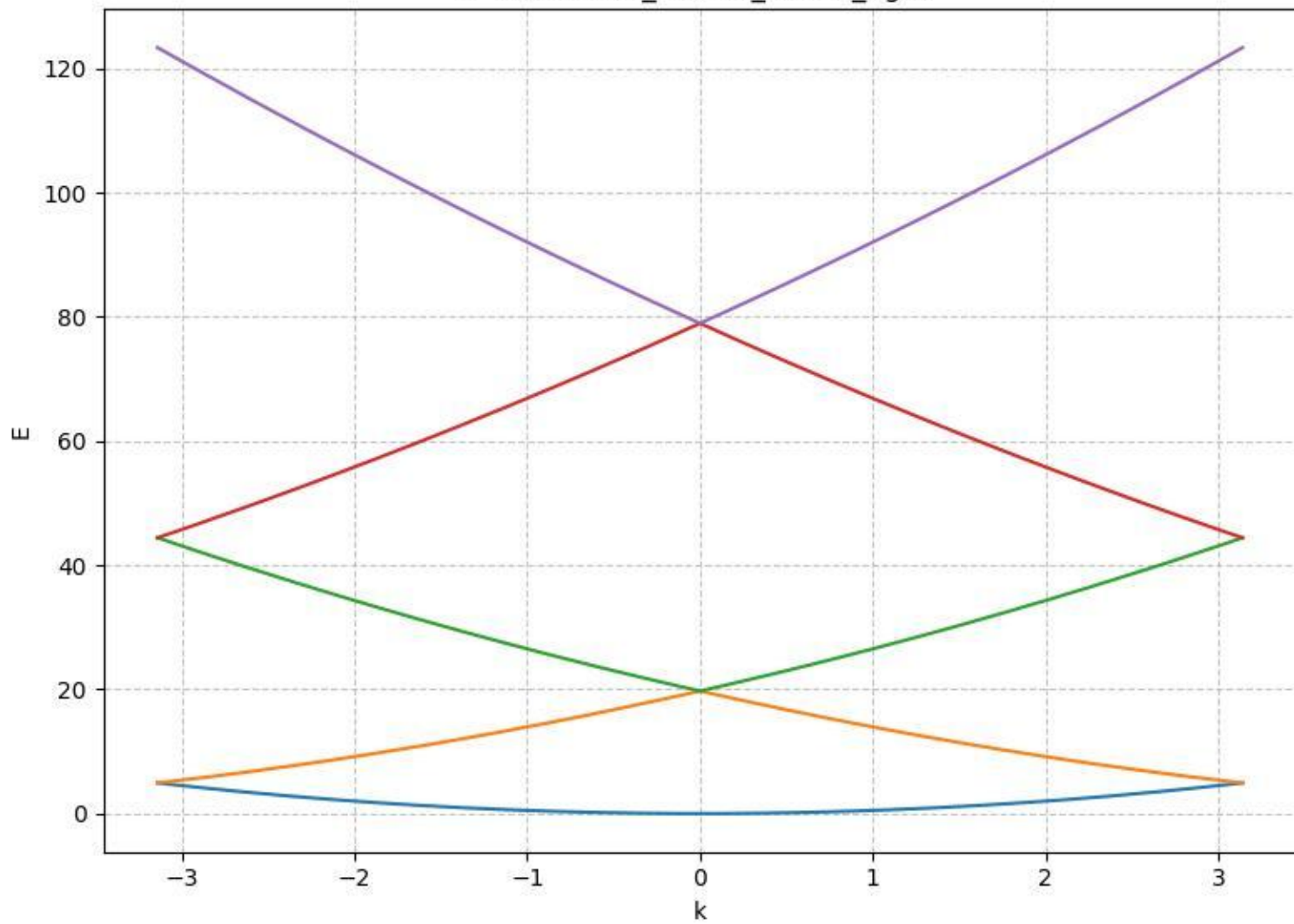
E vs k: a1.00_Vo0.00_nk401_ng61
