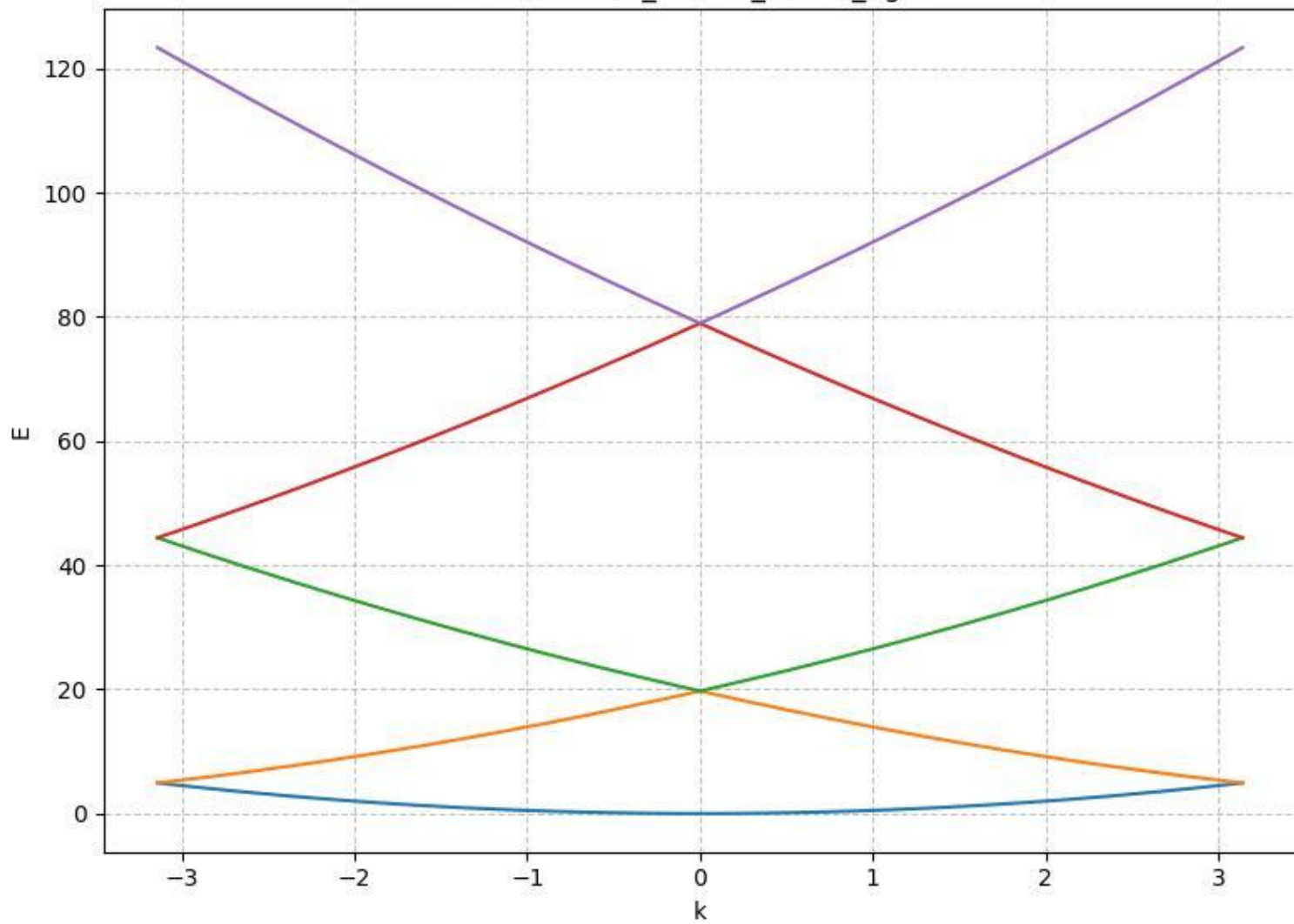
E vs k: a1.00_Vo0.00_nk401_ng11
