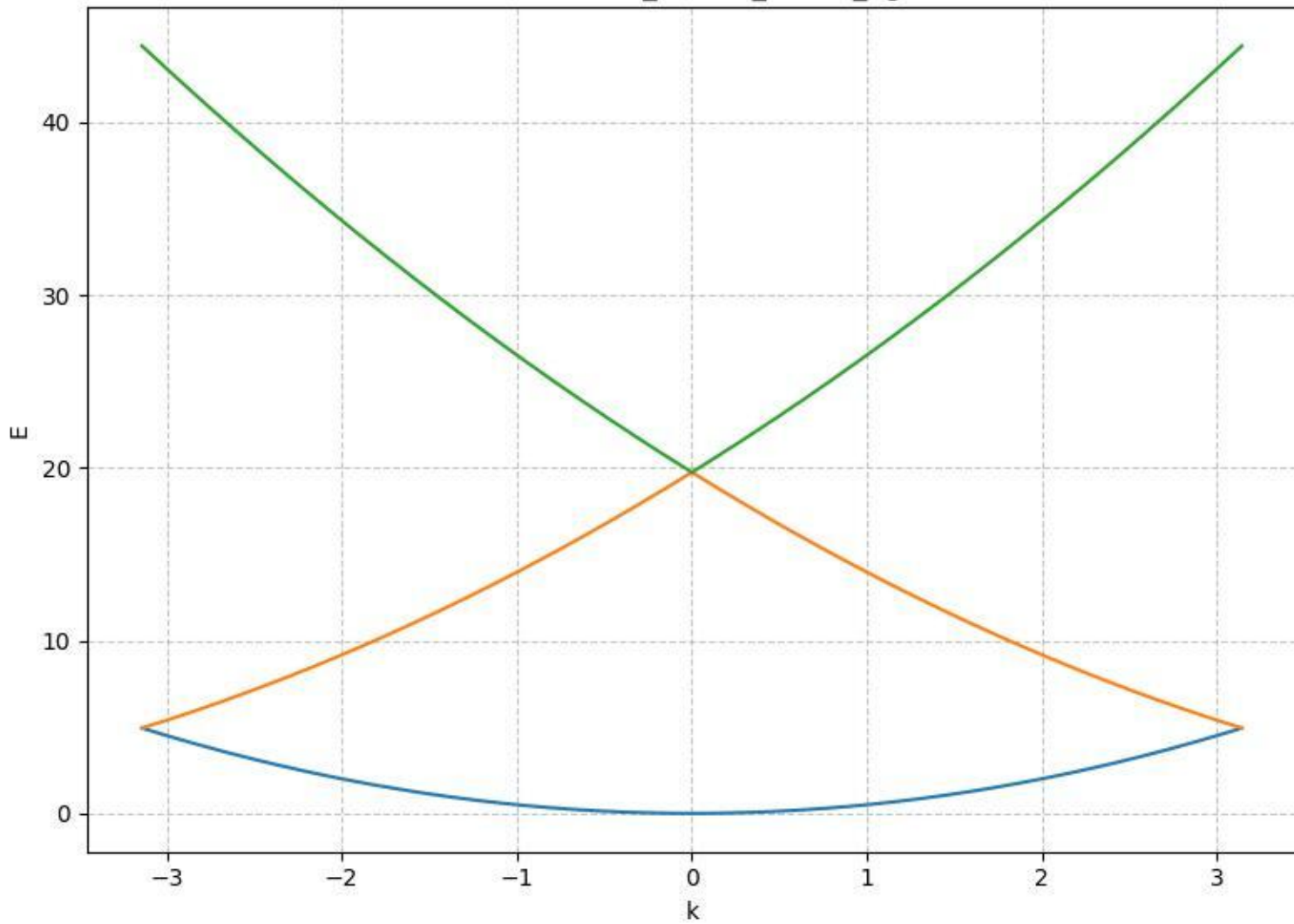
E vs k: a1.00_Vo0.00_nk401_ng3
