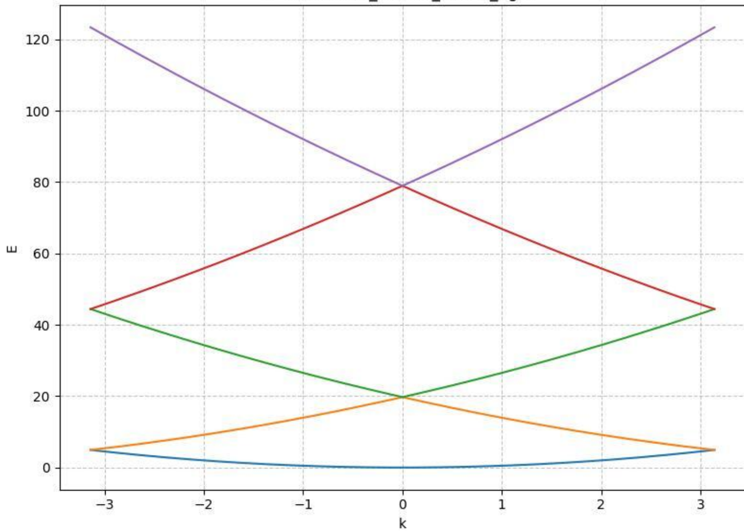
E vs k: a1.00_Vo0.00_nk401_ng21
