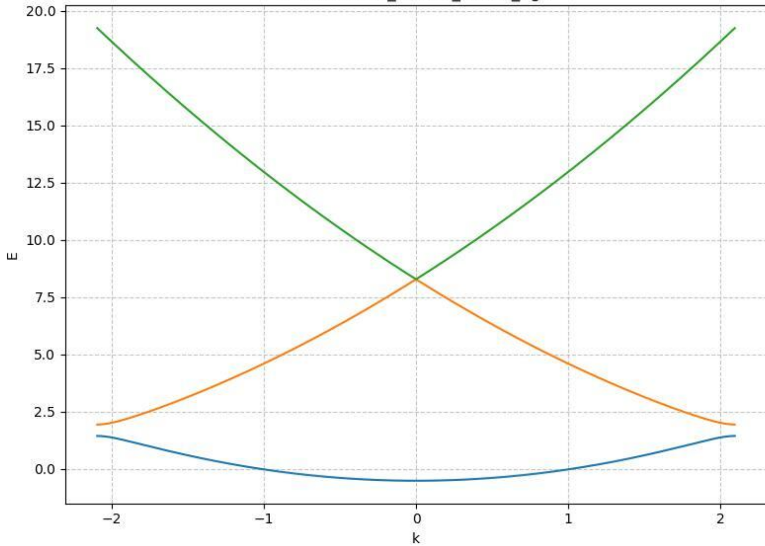
E vs k: a1.50_Vo0.50_nk401_ng3
