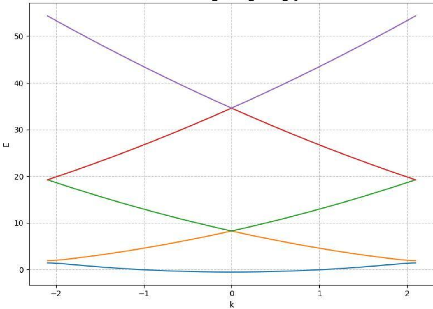
E vs k: a1.50_Vo0.50_nk401_ng21
