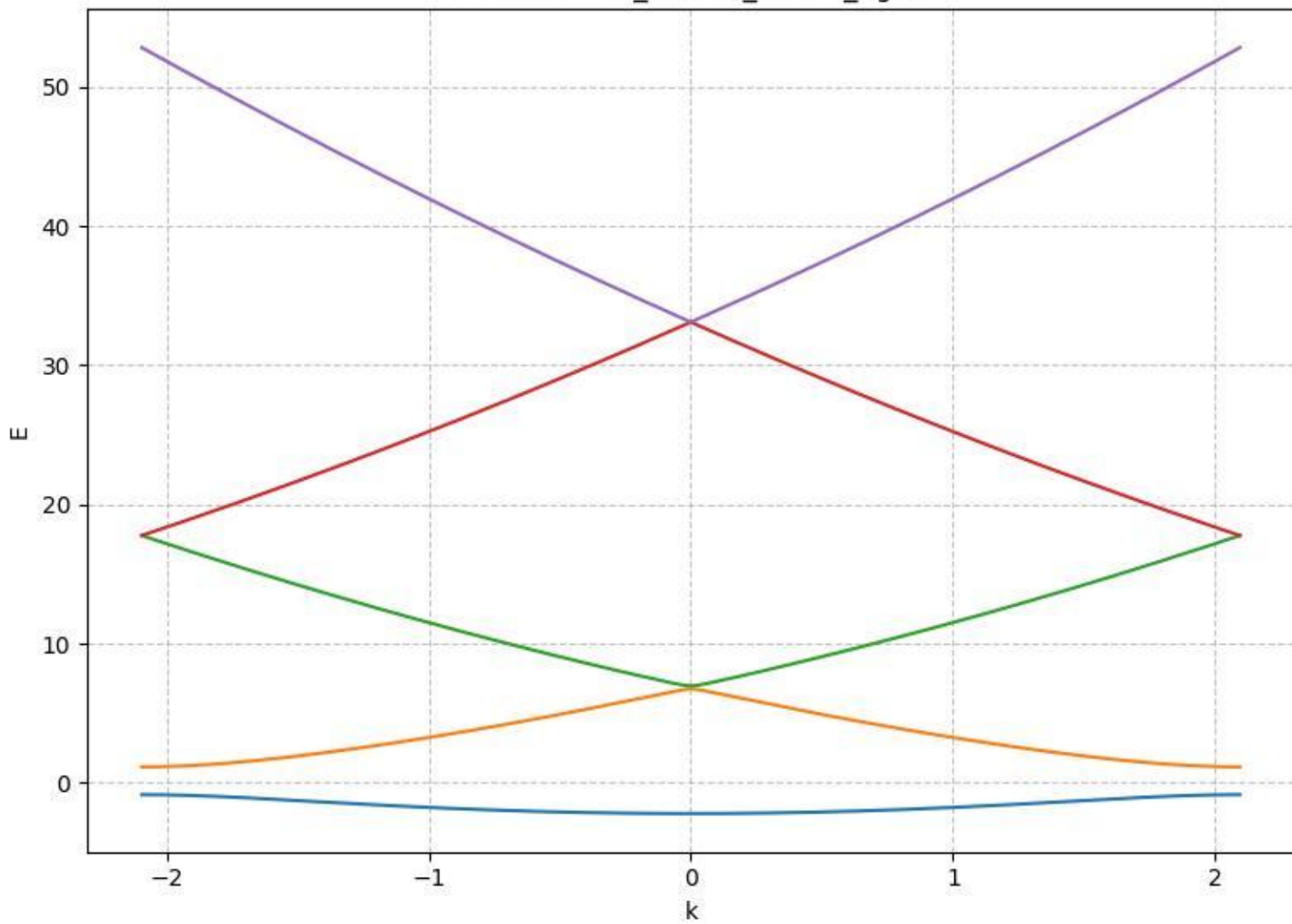
E vs k: a1.50_Vo2.00_nk401_ng21
