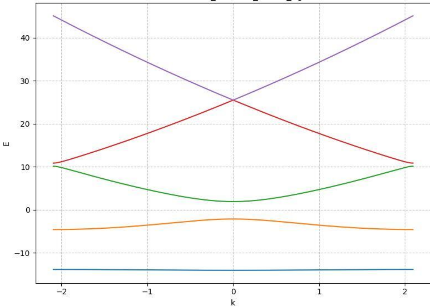
E vs k: a1.50_Vo10.00_nk401_ng21
