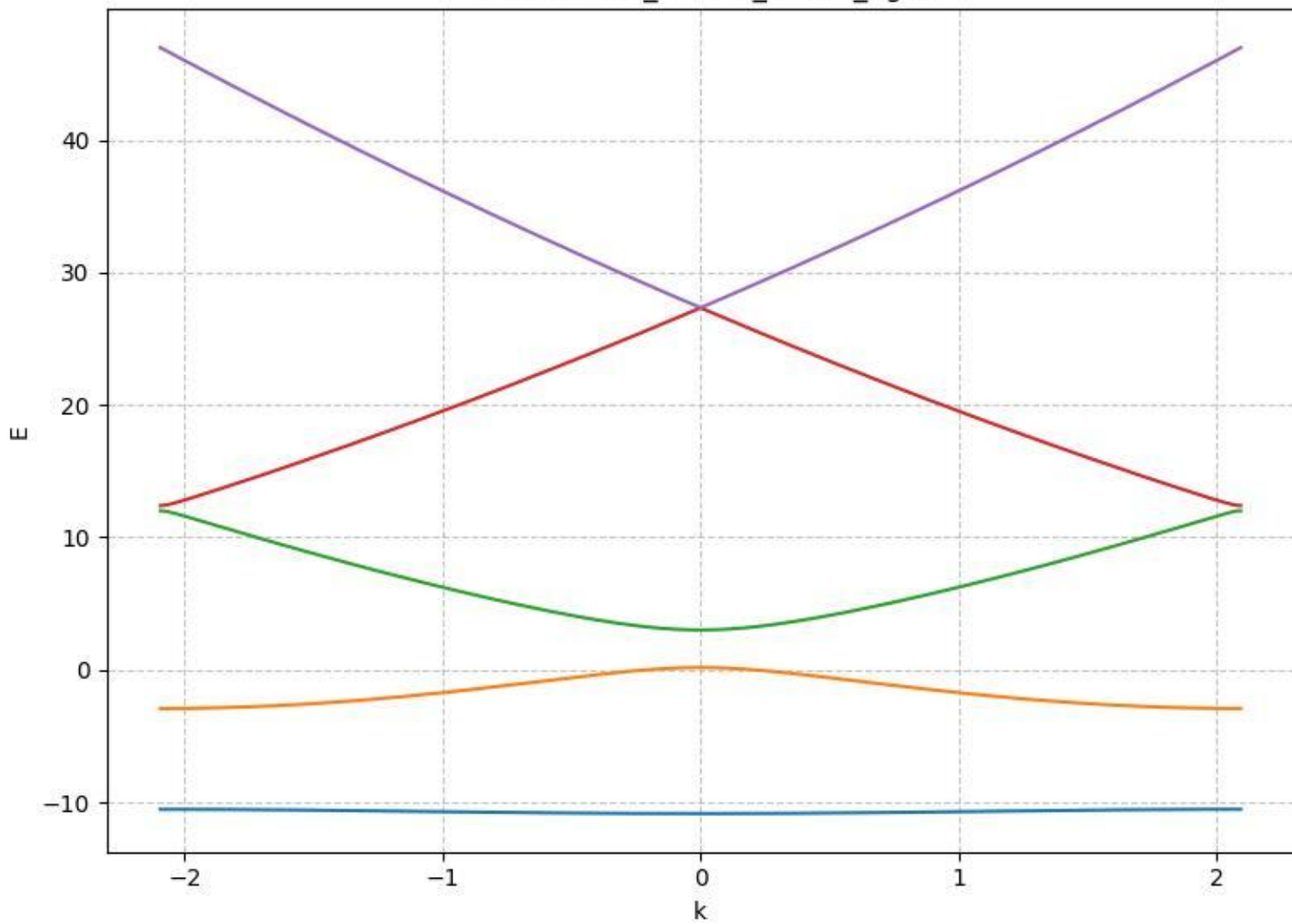
E vs k: a1.50_Vo8.00_nk401_ng21
