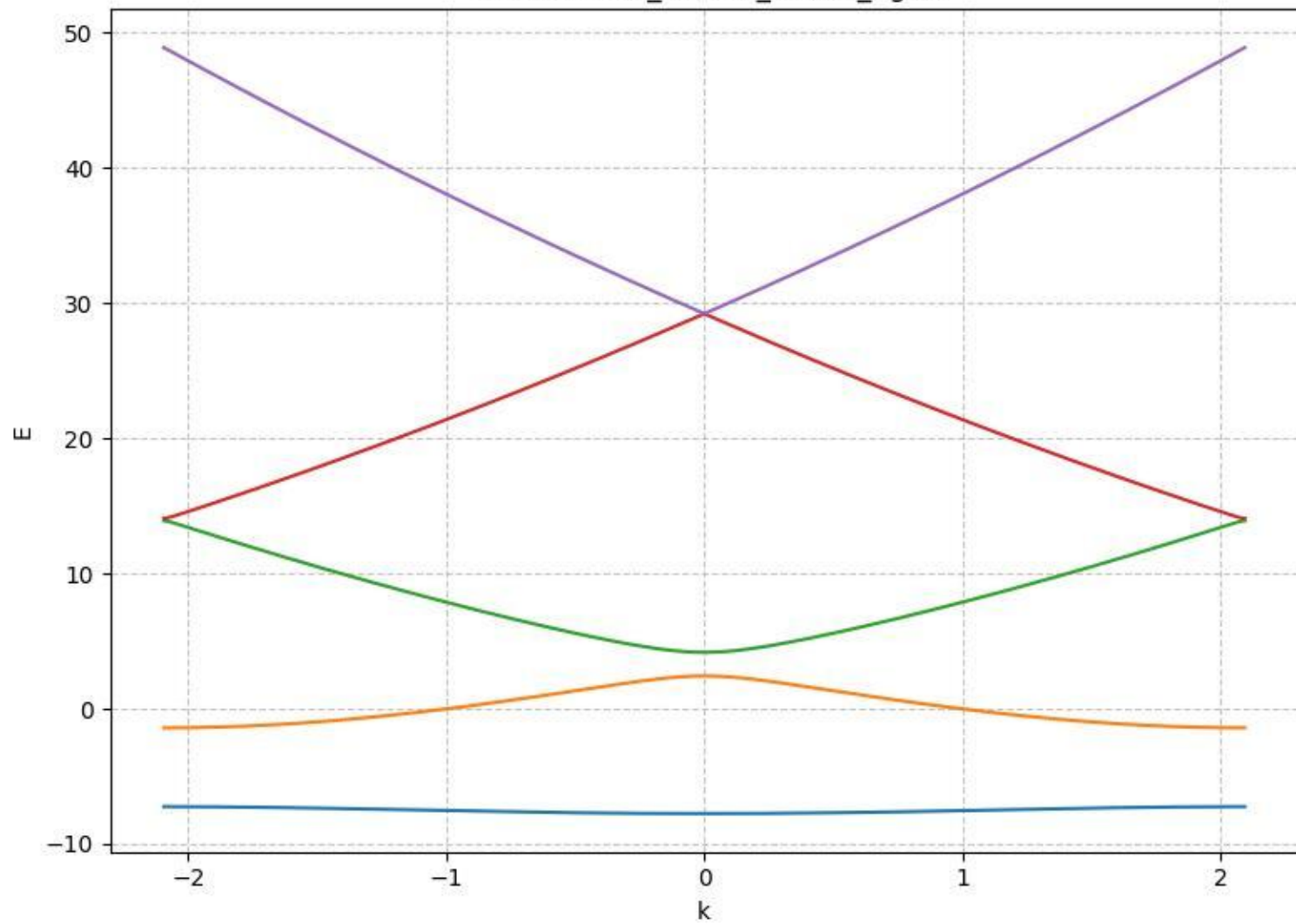
E vs k: a1.50_Vo6.00_nk401_ng21
