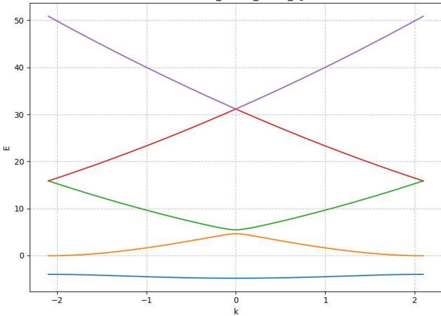
E vs k: a1.50_Vo4.00_nk401_ng21
