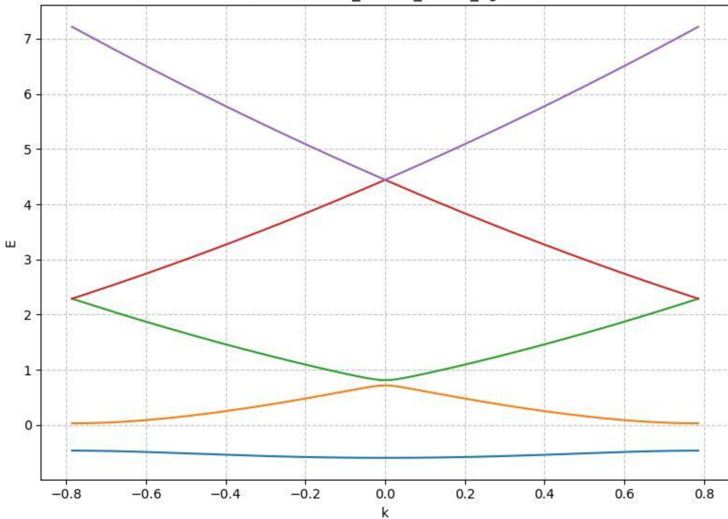
E vs k: a4.00_Vo0.50_nk401_ng21
