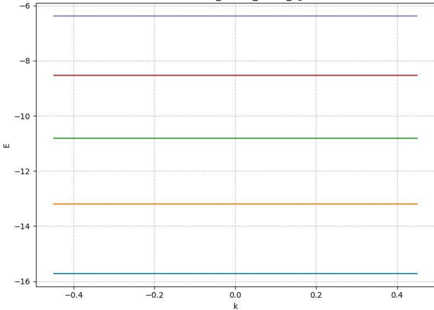
E vs k: a7.00_Vo8.50_nk401_ng21
