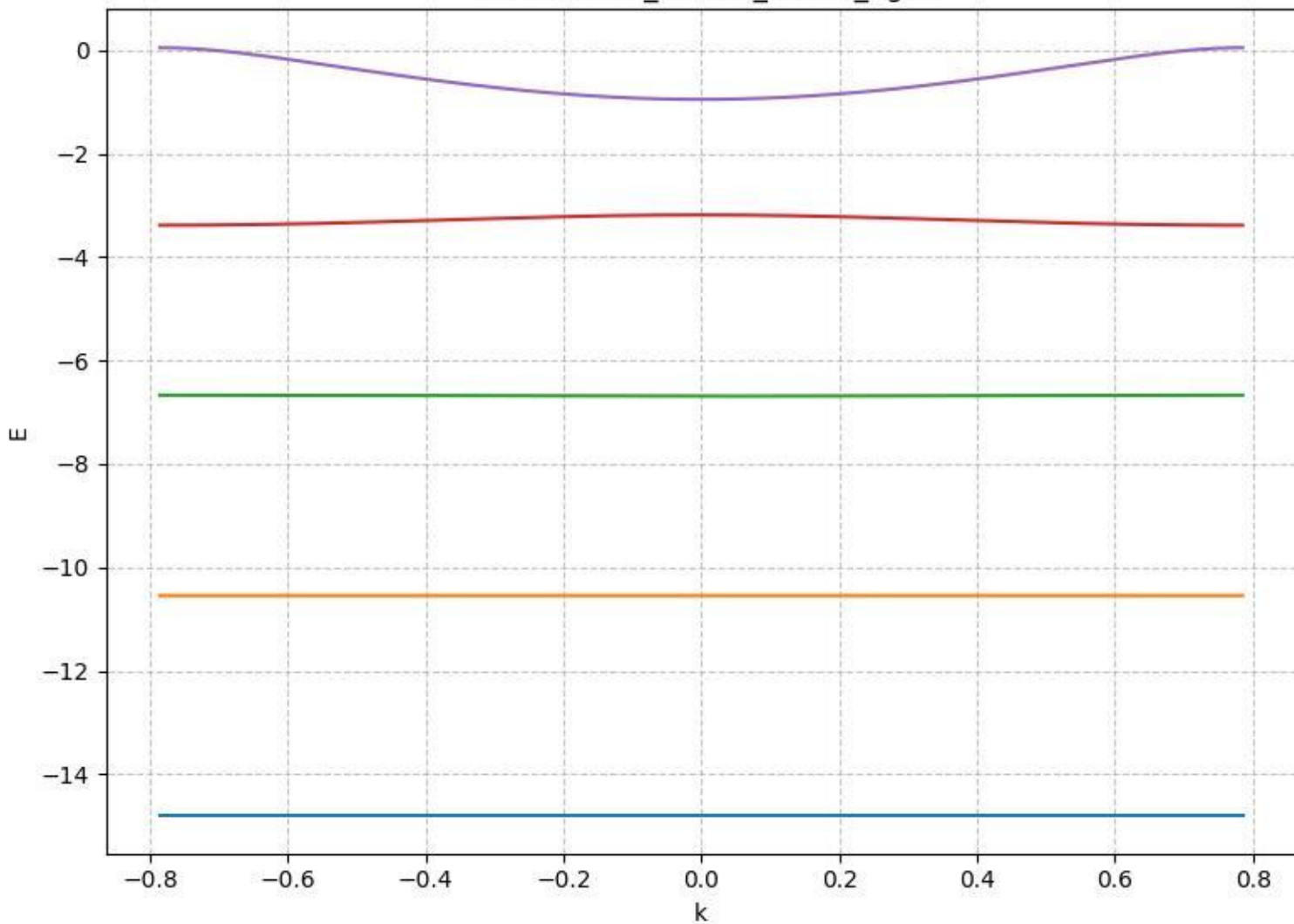
E vs k: a4.00_Vo8.50_nk401_ng21
