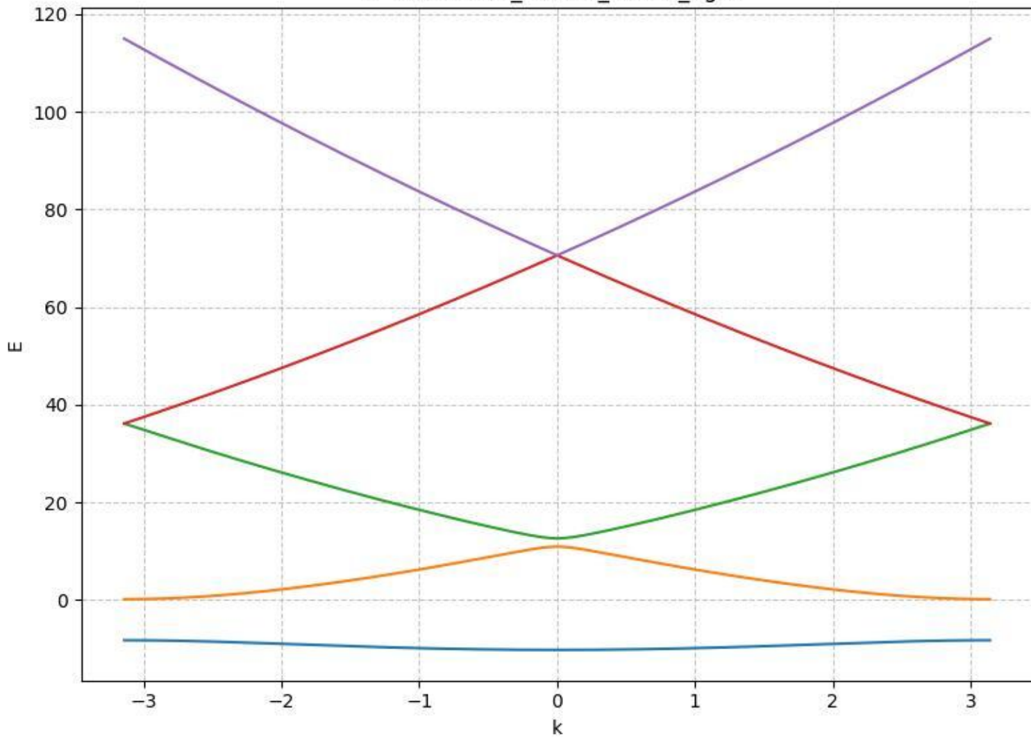
E vs k: a1.00_Vo8.50_nk401_ng21
