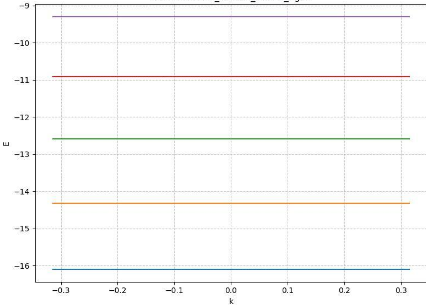
E vs k: a10.00_Vo8.50_nk401_ng21
