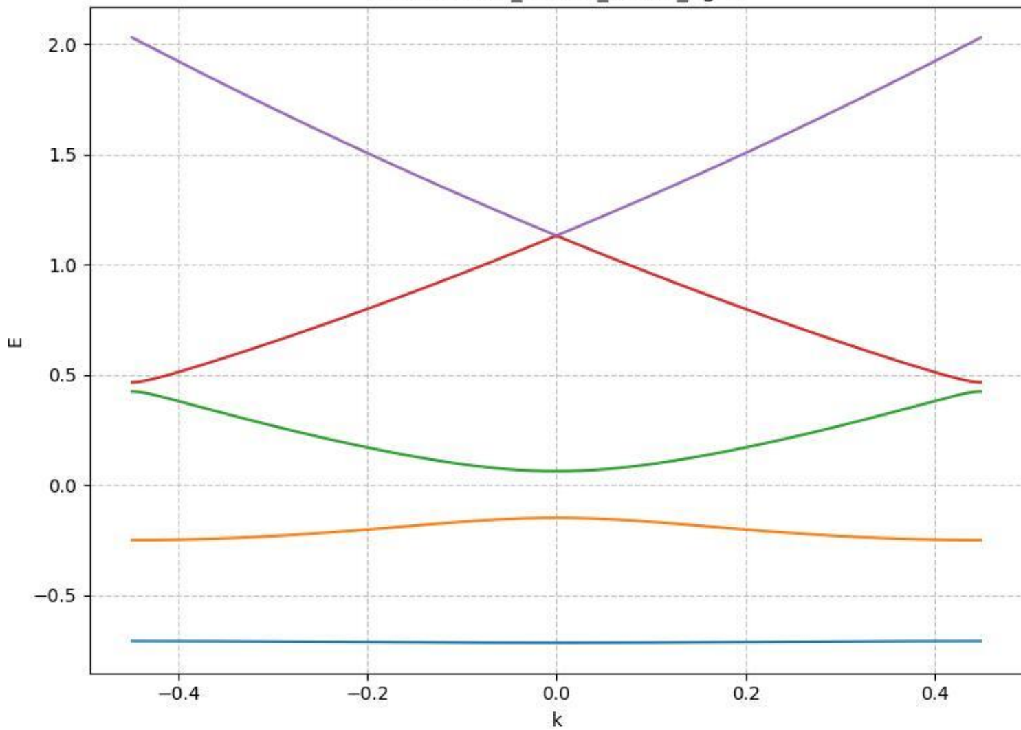
E vs k: a7.00_Vo0.50_nk401_ng21
