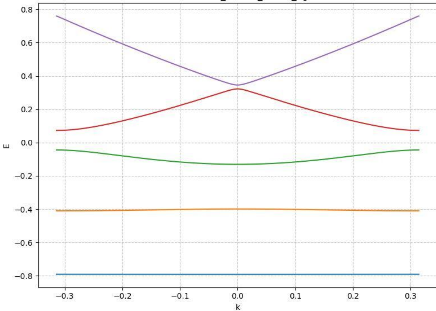
E vs k: a10.00_Vo0.50_nk401_ng21
