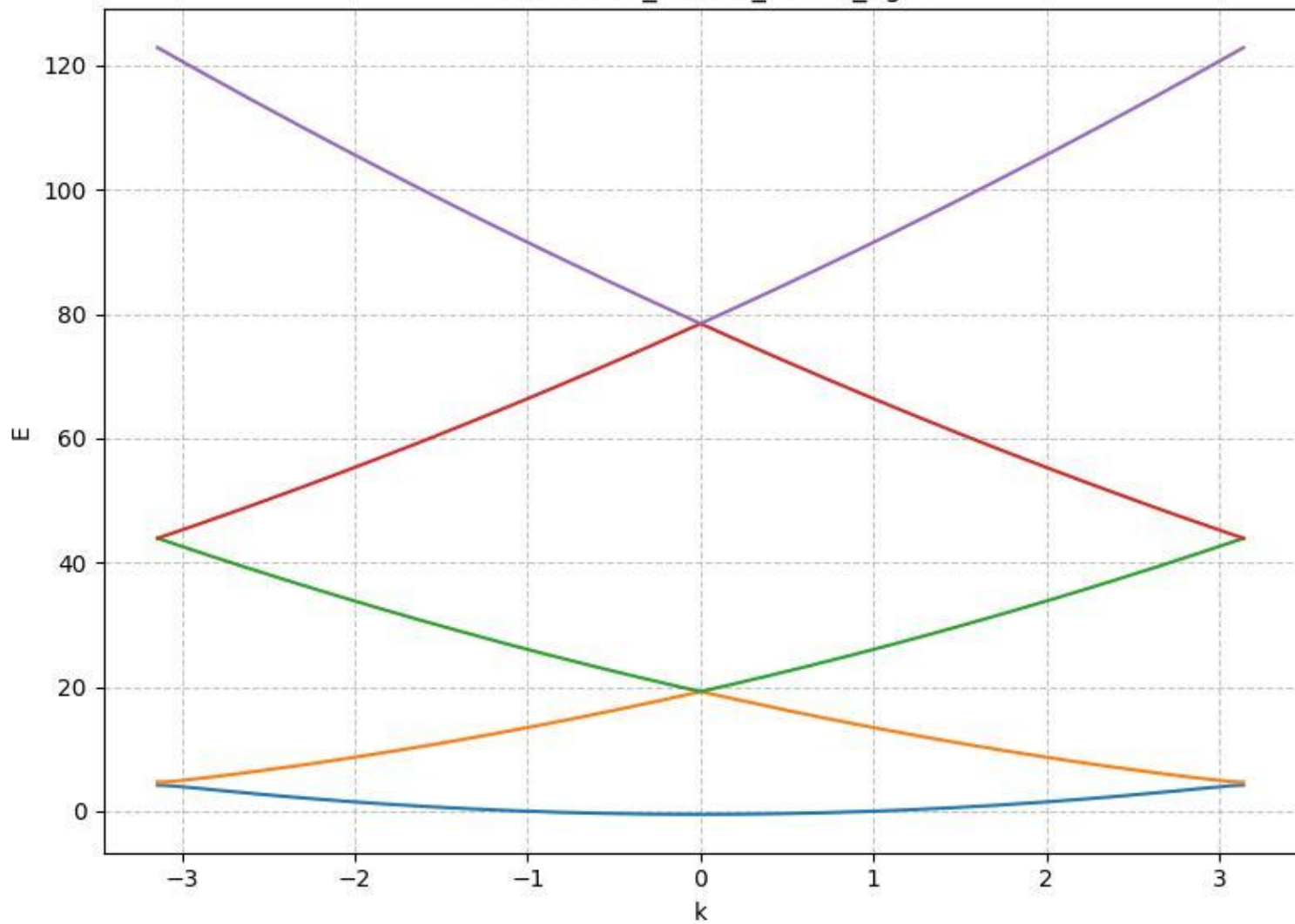
E vs k: a1.00_Vo0.50_nk401_ng21
