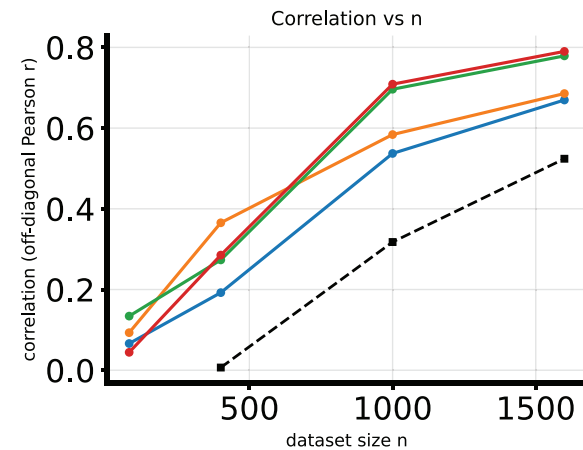
fourier input
