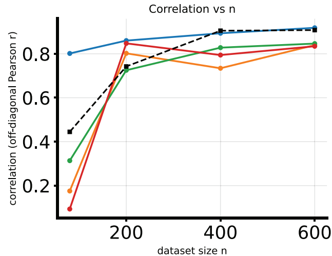
Fourier input
