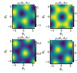
fourier input
