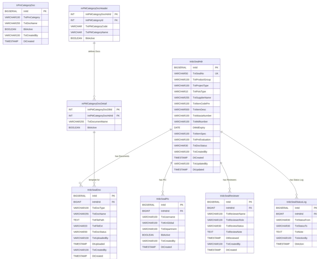
ERD – Relasi Tabel Modul SEAL
