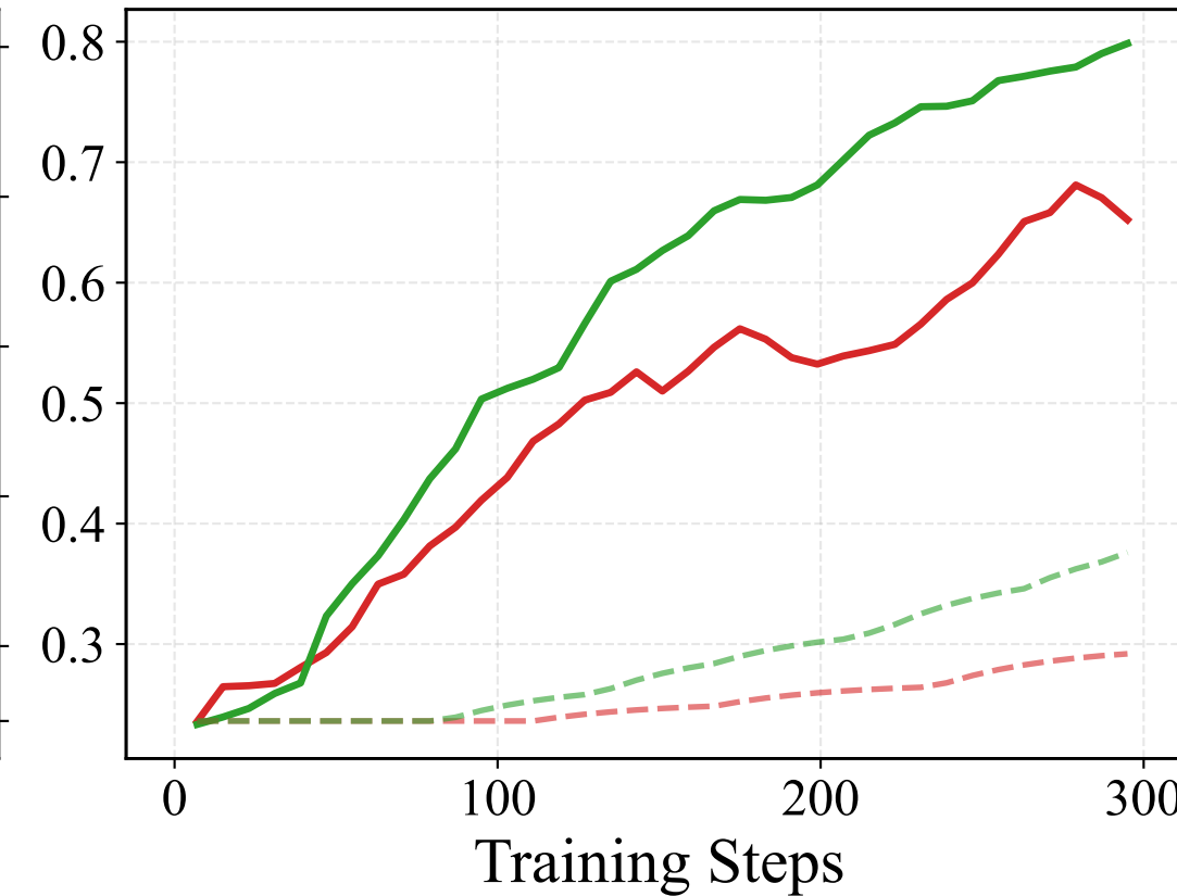
BSTAudit
