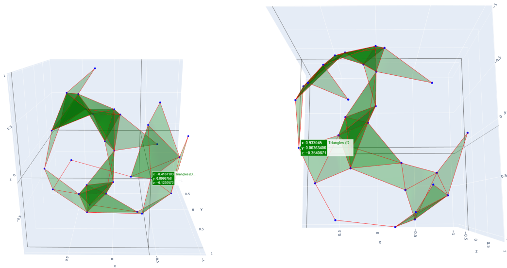
Σχήμα 5: Οπτικοποίηση του συμπλέγματος σε 3 διαστάσεις (3D) για τον Τόρο από δύο διαφορετικές οπτικές γωνίες.
