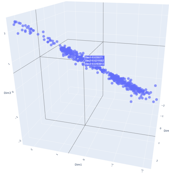
Σχήμα 15: Τρισδιάστατη τροχιά του Takens Embedding ( d = 3, \tau = 1 ) για τη χρονοσειρά S&P 500.
