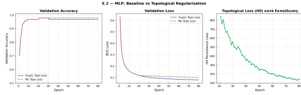
Σχήμα 20: Training curves του Validation και εξέλιξη του Topological Loss.
