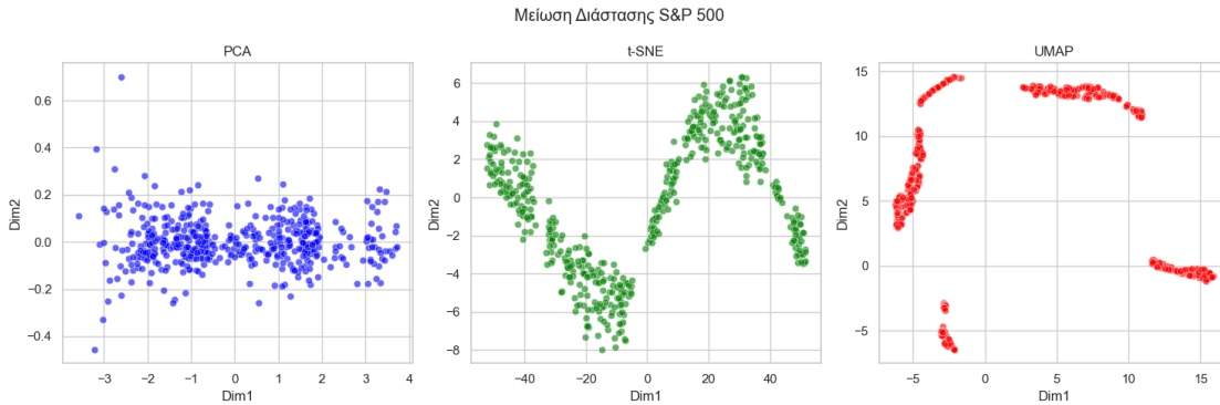
Σχήμα 17: Σύγκριση μείωσης διάστασης του 3D Takens Embedding του S&P 500 με PCA, t-SNE και UMAP.
