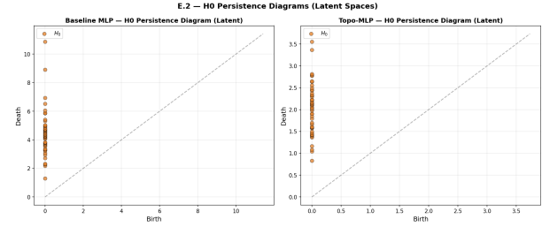
Σχήμα 23: H_0 Persistence Diagrams των αντίστοιχων latent spaces.
