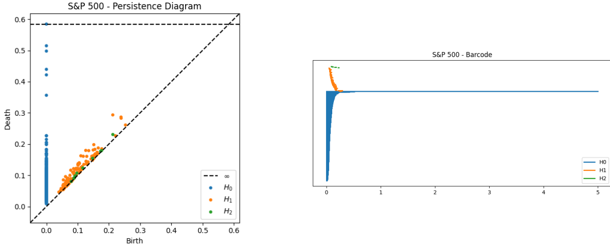
Σχήμα 15: Persistence Diagram (αριστερά) και Barcode (δεξιά) για το point cloud της χρονοσειράς Σ&Π 500.
