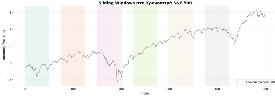
Σχήμα 18: Sliding windows στη χρονοσειρά S&P 500 που χρησιμοποιήθηκαν για την κατασκευή των point clouds.
