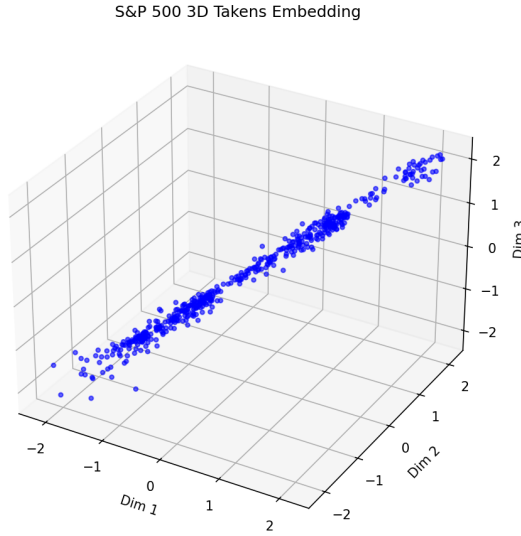
Σχήμα 16: Τριδιάστατη τροχιά του Takens Embedding ( d = 3, \tau = 1 ) για τη χρονοσειρά S&P 500.
