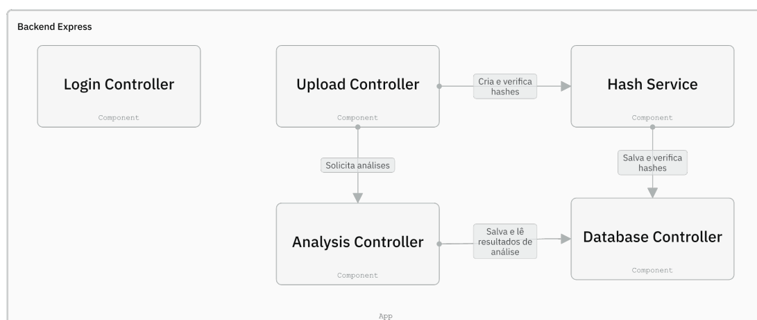
Figura 6 – C4 Model — Nível 3 (Componentes do Backend Express).
