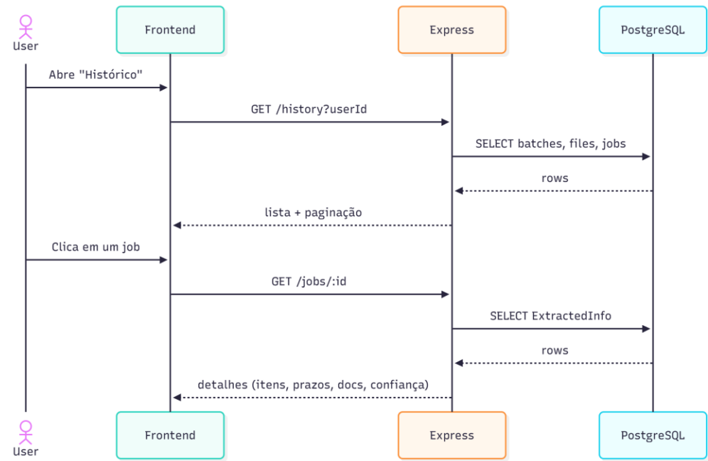
Fluxograma do Sistema Hash
