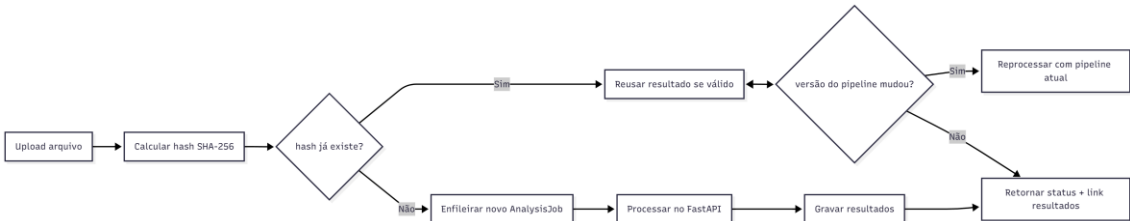
Fluxograma do Sistema Hash
