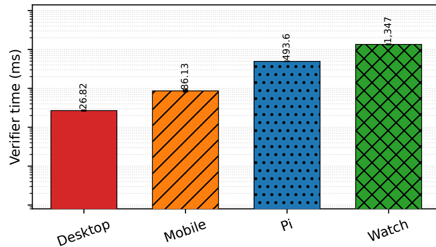
bbs2023(JS)
