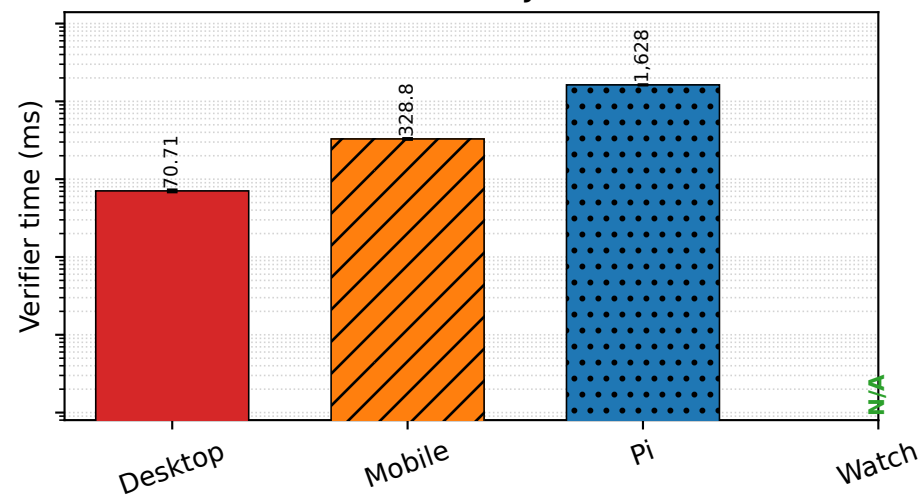
bbs2023(JS)
