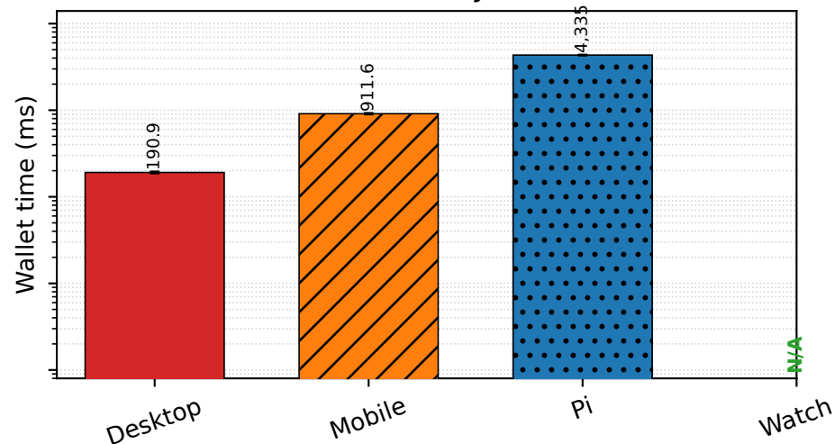
bbs2023(JS)
