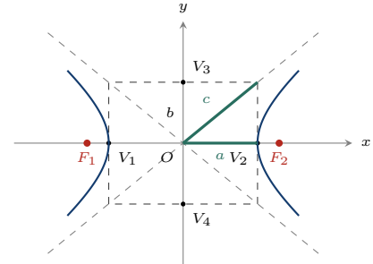
Figura 2.2: Elementos da Hipérbole.
