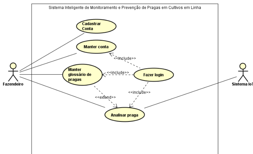
Figura 3 – Diagrama de Caso de Uso do AGRO-G.E.S.F.
