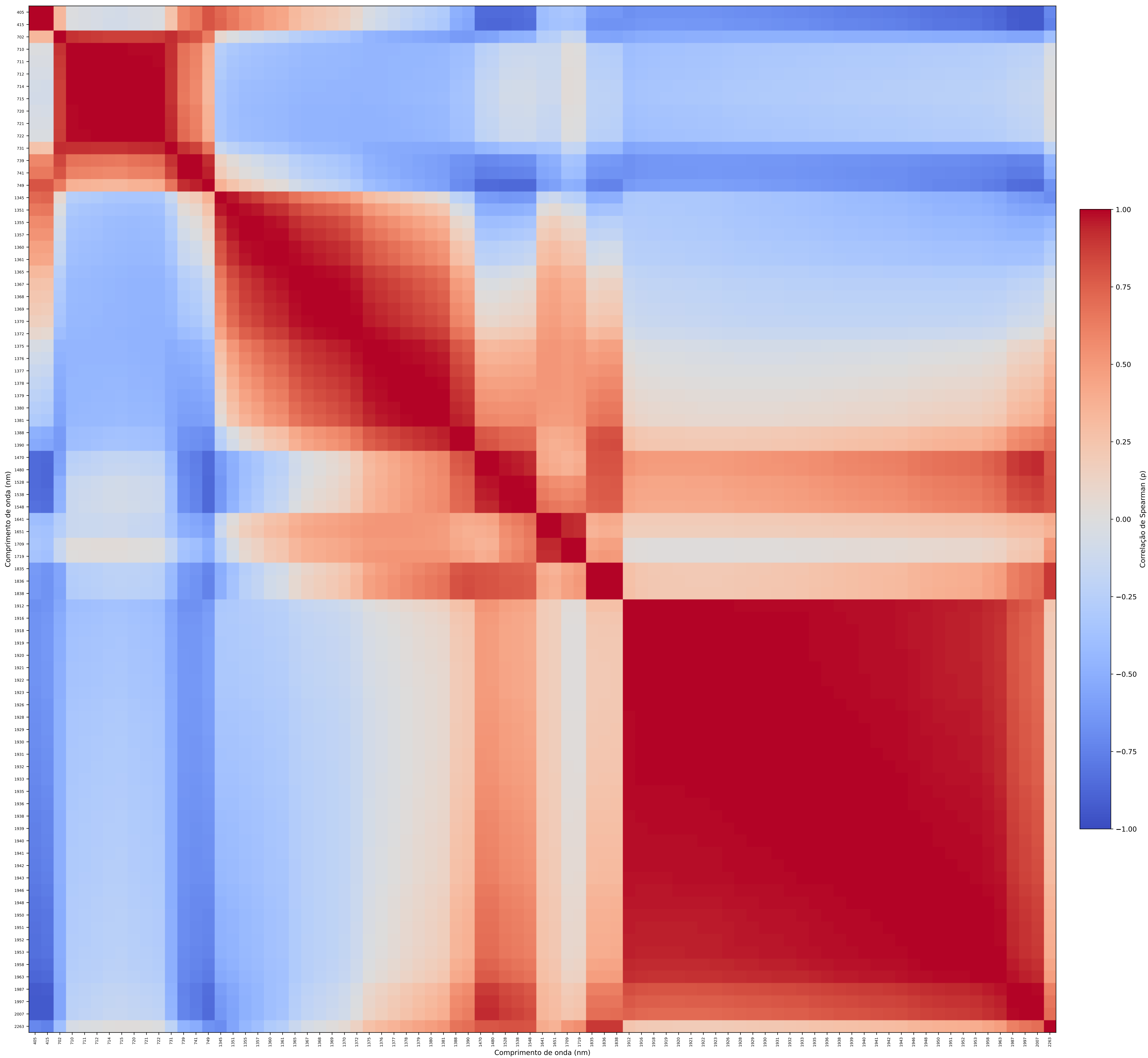
Correlograma consolidado: união das Top 5 VIP de todos os genótipos e dias Spearman; todas as leituras da manhã
