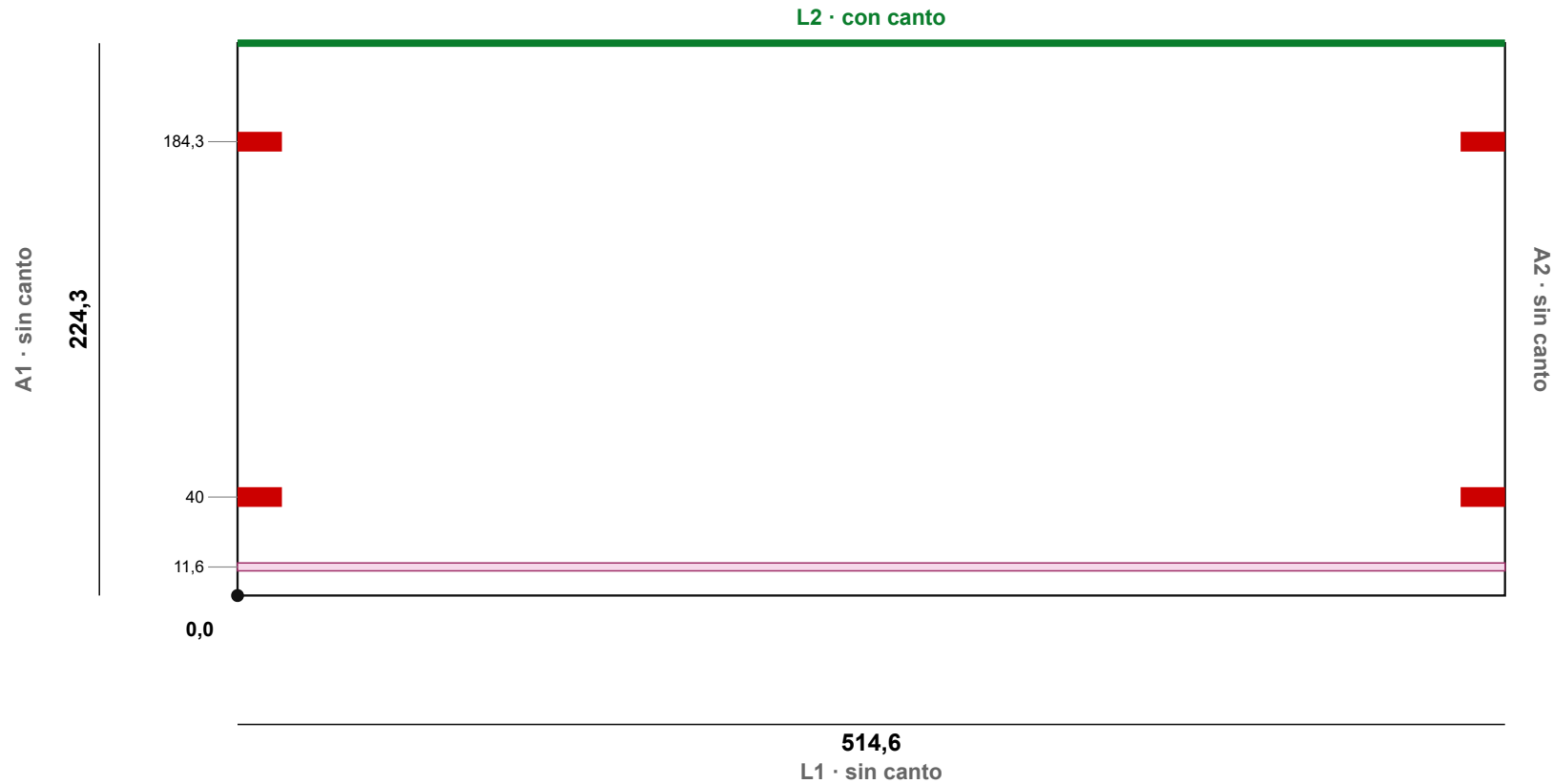
Perforaciones de canto (centradas en el espesor)
