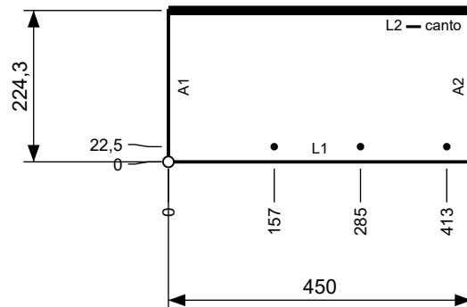
Cara A · escala 1:10
