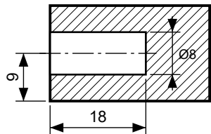
Detalle B — perforación de canto (esc. 1:1)
