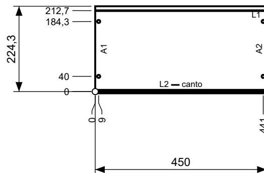
Cara B (pieza dada vuelta) · escala 1:10
