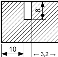
Detalle C — ranura cara A (esc. 1:1)
