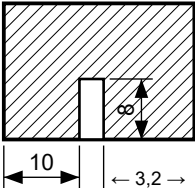
Detalle A — ranura cara B (esc. 1:1) medida desde el canto L1
