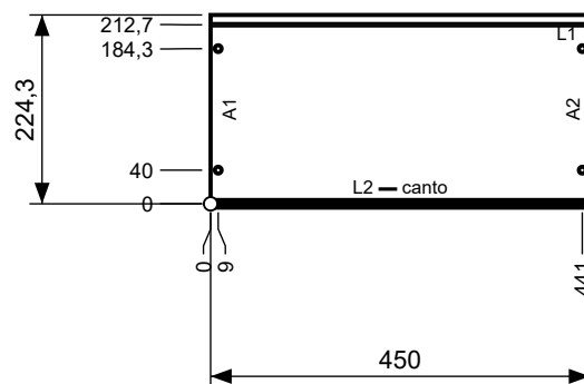
Cara B (pieza dada vuelta) · escala 1:10
