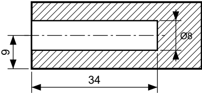
Detalle A — perforación de canto (esc. 1:1)
