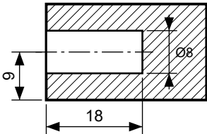
Detalle A — perforación de canto (esc. 1:1)
