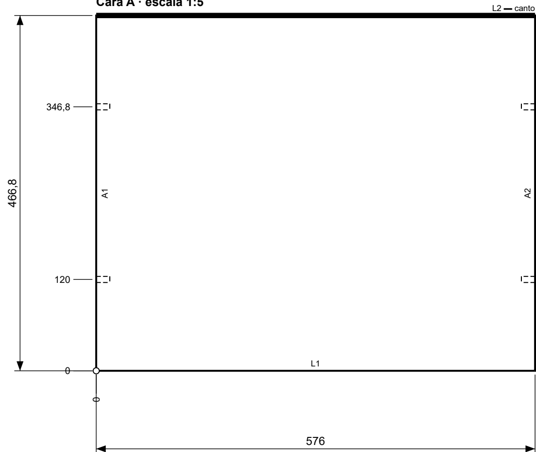
Cara A · escala 1:5
