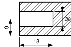
Detalle A — perforación de canto (esc. 1:1)
