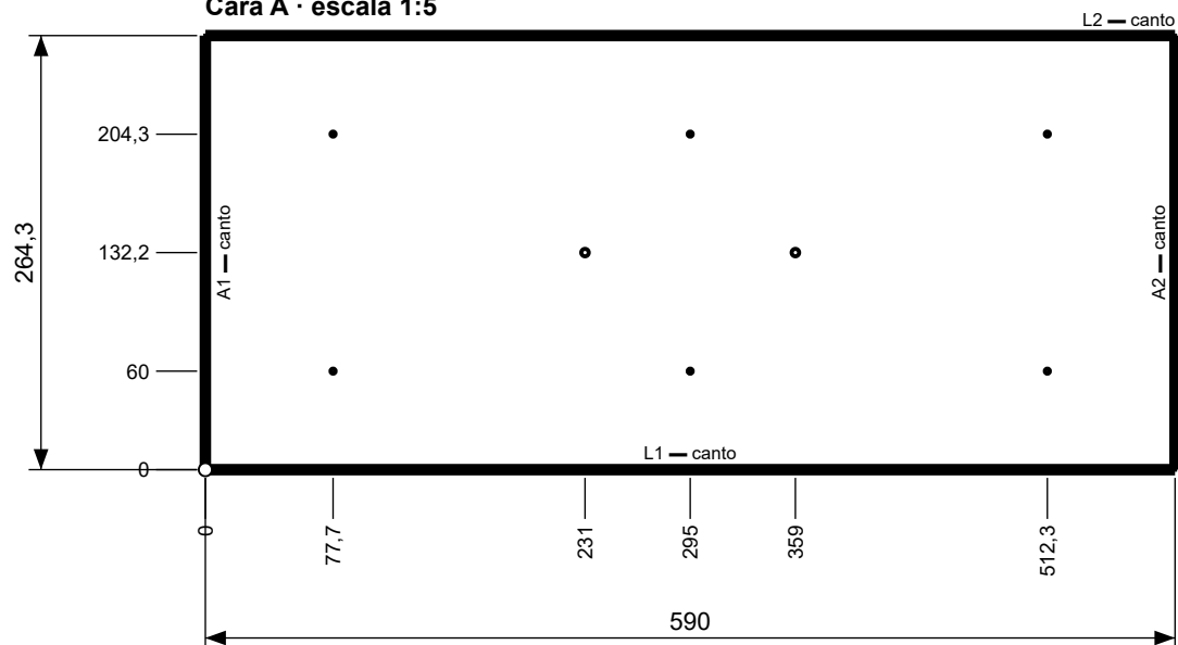
Cara A · escala 1:5
