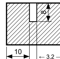
Detalle B — ranura cara A (esc. 1:1)
