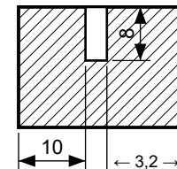
Detalle A — ranura cara A (esc. 1:1)
