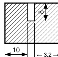
Detalle A — ranura cara A (esc. 1:1)
