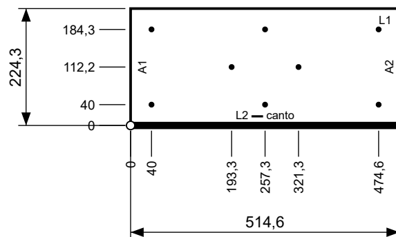
Cara B — pieza dada vuelta de arriba hacia abajo · escala 1:10
