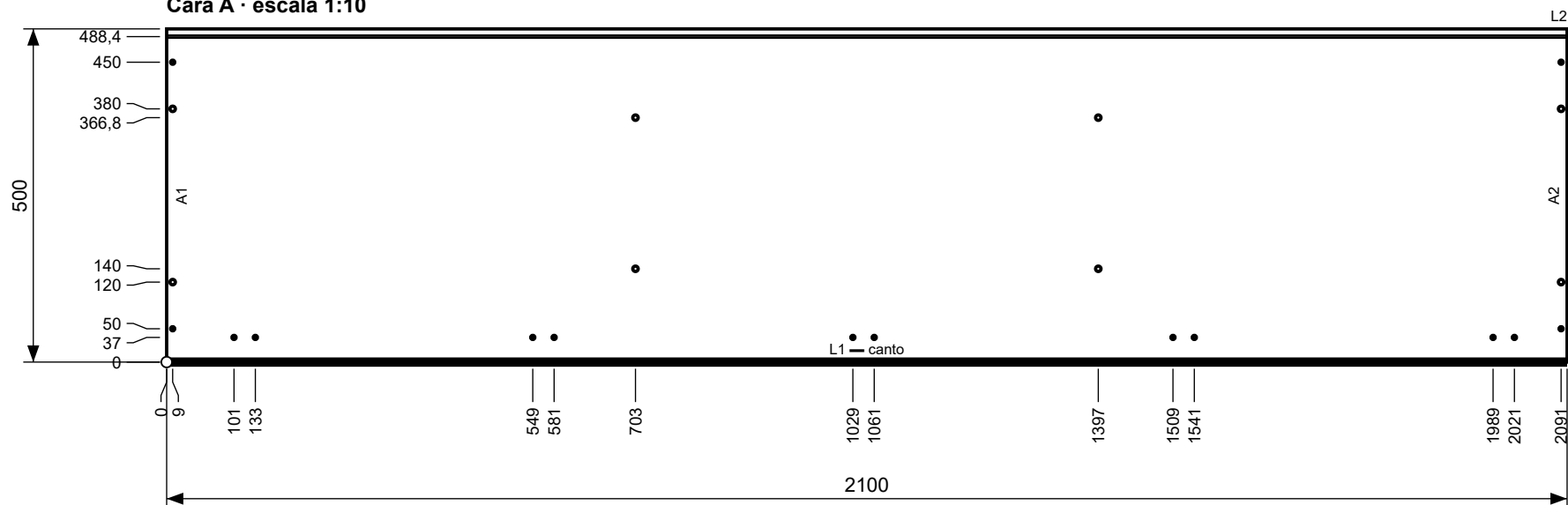
Cara A · escala 1:10
