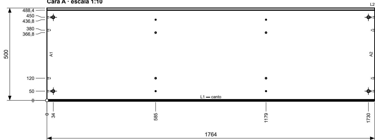
Cara A · escala 1:10
