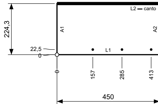
Cara A · escala 1:10
