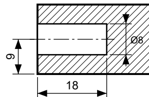
Cara B — pieza dada vuelta de arriba hacia abajo · escala 1:10
