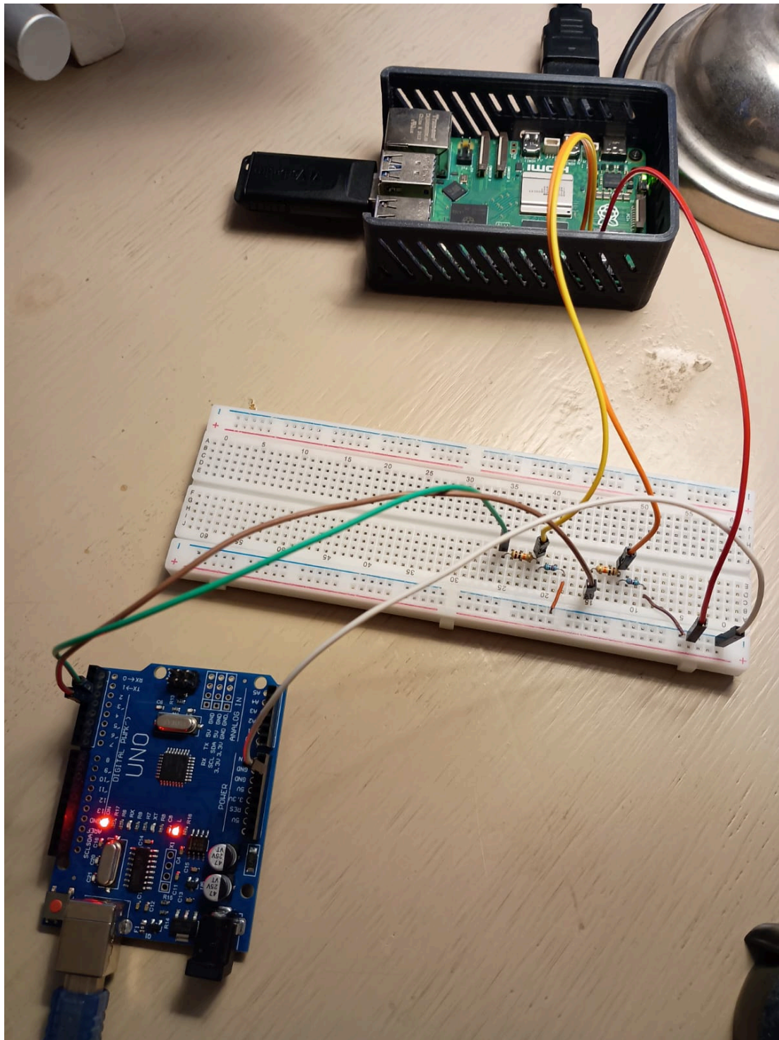
1.2: Circuito físico utilizado para generar y leer las señales digitales
