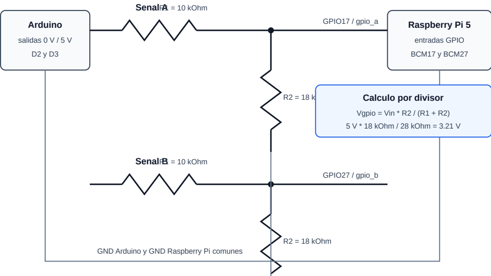
1.3: Divisores resistivos usados para adaptar las señales del Arduino a GPIO de Raspberry Pi
