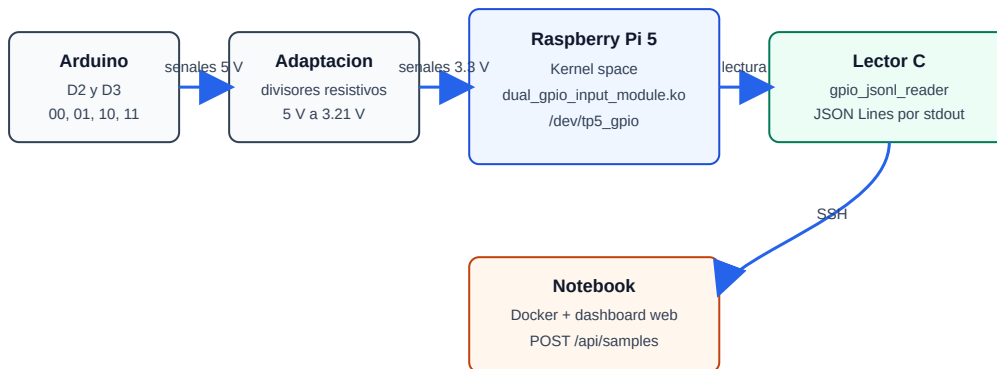
1.1: Diagrama de bloques del flujo Arduino, Raspberry Pi, SSH y dashboard web
