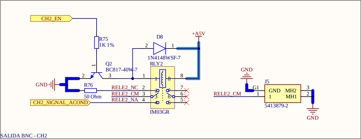
SALIDA BNC - CH2
