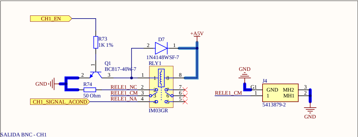
SALIDA BNC - CH1
