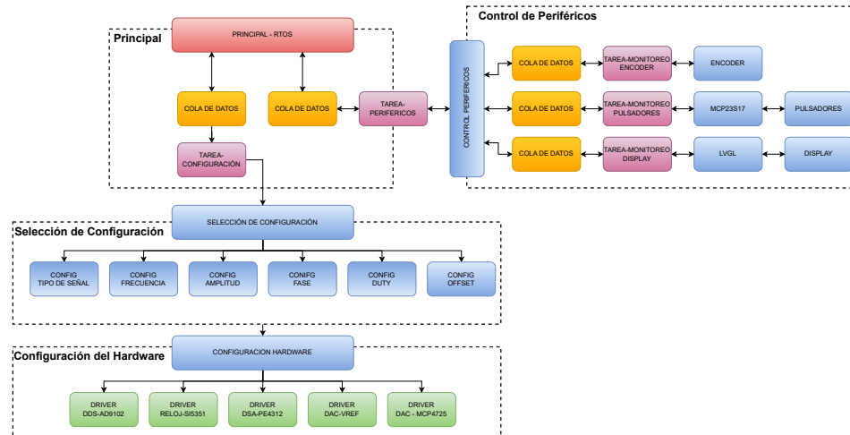
Figura 8: Diagrama en bloques del firmware.
