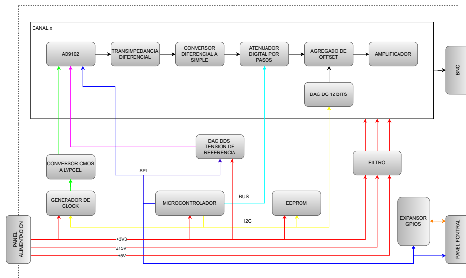
Figura 6: Diagrama en bloques del Hardware del Generador de Funciones Arbitrarias de la Placa de Control.
