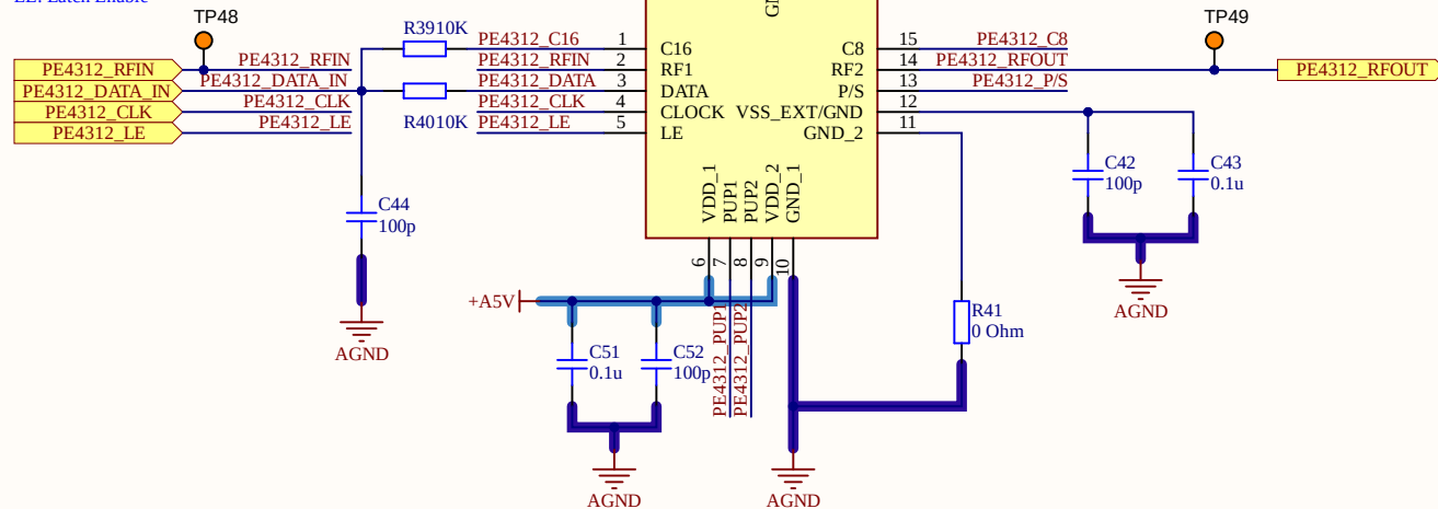
ATENUADOR DIGITAL POR PASOS PE4312
