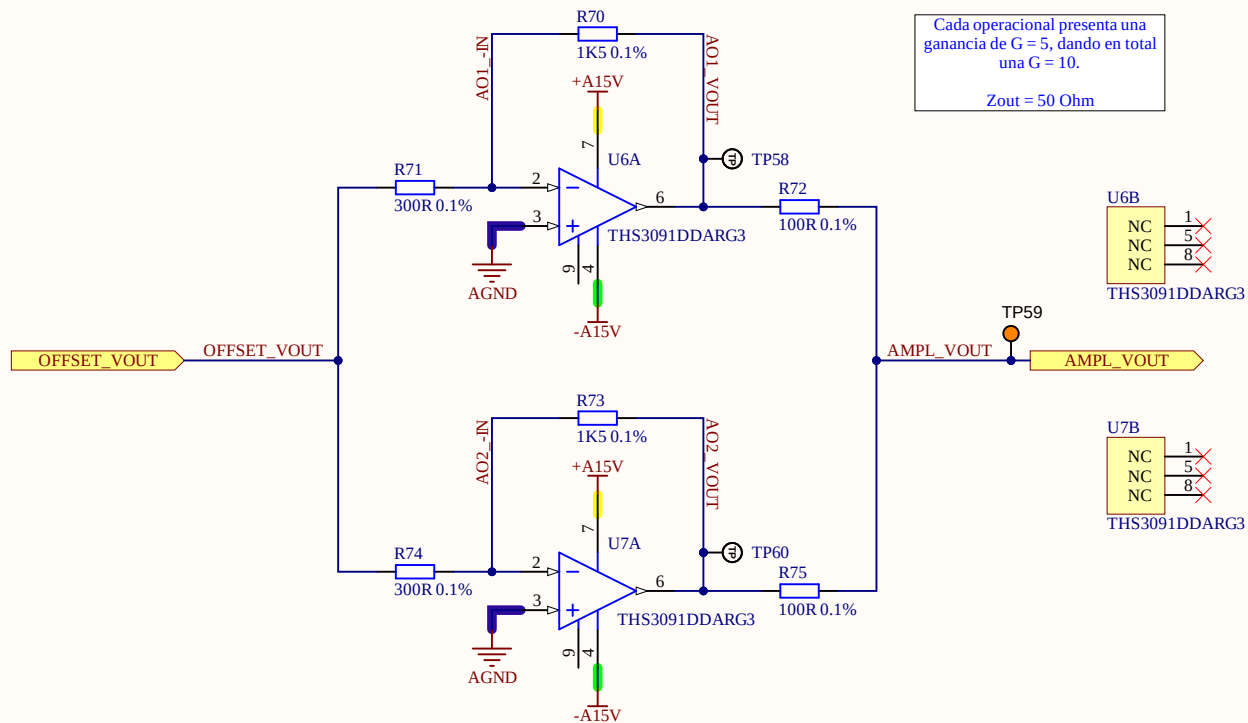
AMPLIFICADOR PRINCIPAL-SALIDA 50 OHM
