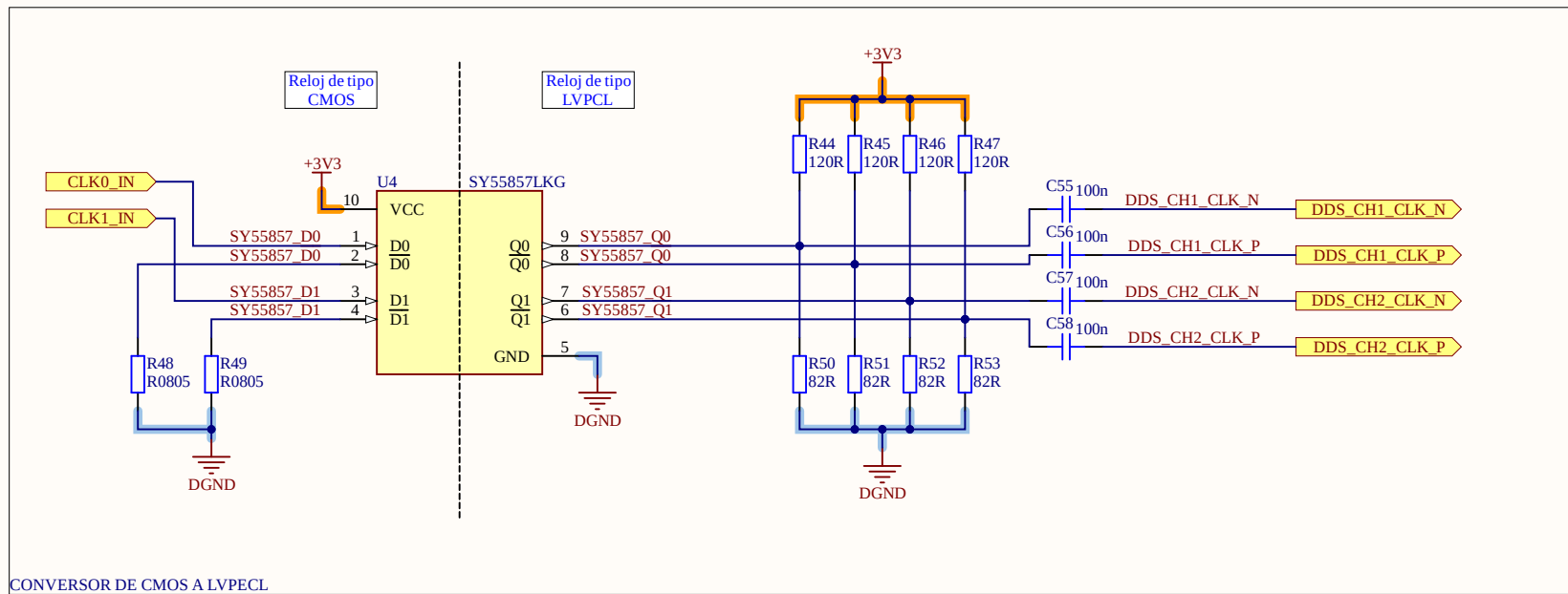
CONVERSOR DE CMOS A LVPECL
