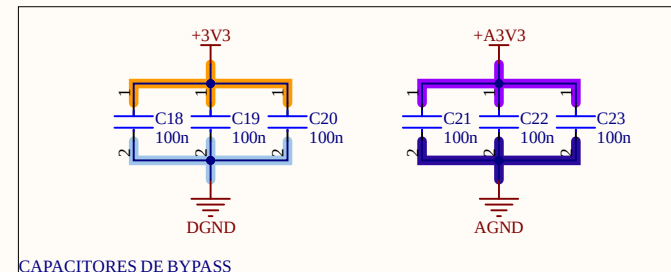
CAPACITORES DE BYPASS
