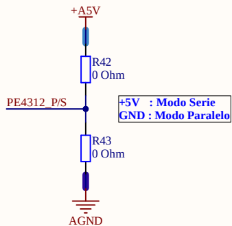
CONFIGURACION MODO PARALELO/SERIAL
