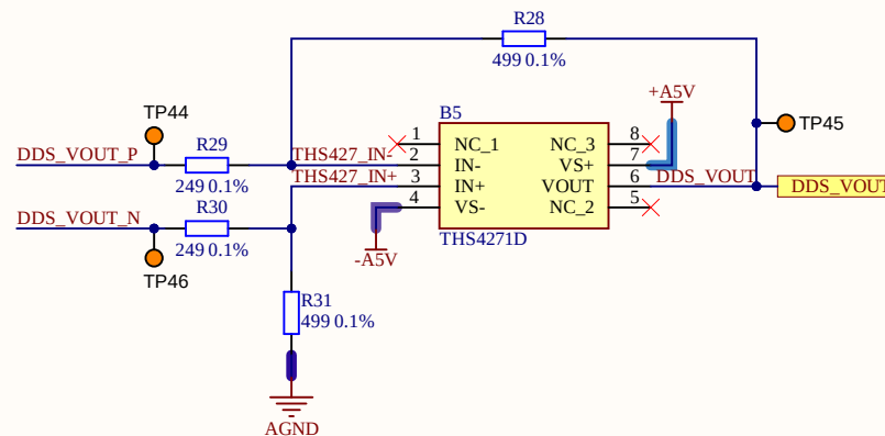
AMPLIFICADOR RESTADOR
