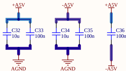
CAPACITORES DE BYPASS
