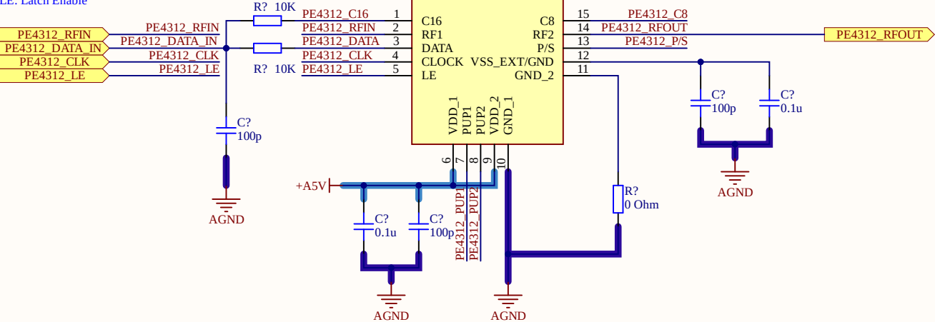
ATENUADOR DIGITAL POR PASOS PE4312
