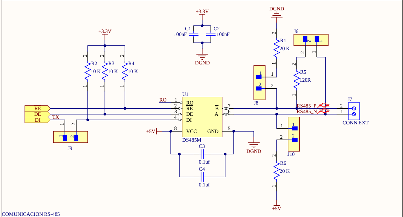
COMUNICACION RS-485
