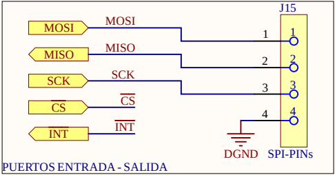
PUERTOS ENTRADA - SALIDA
