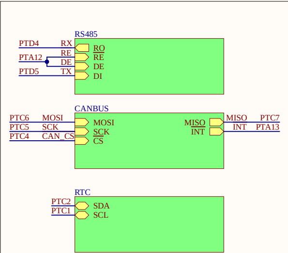
COMUNICACIONES
