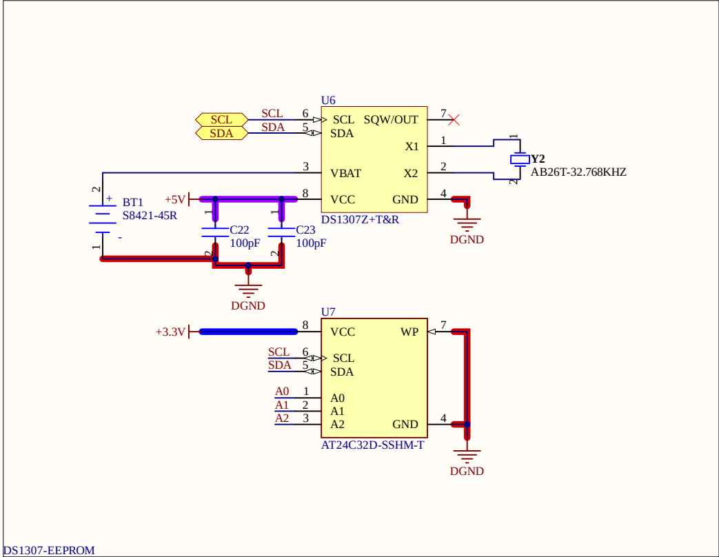
DS1307-EEPROM
