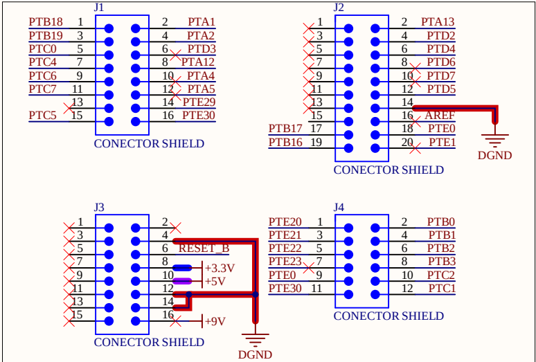
CONECTORES
