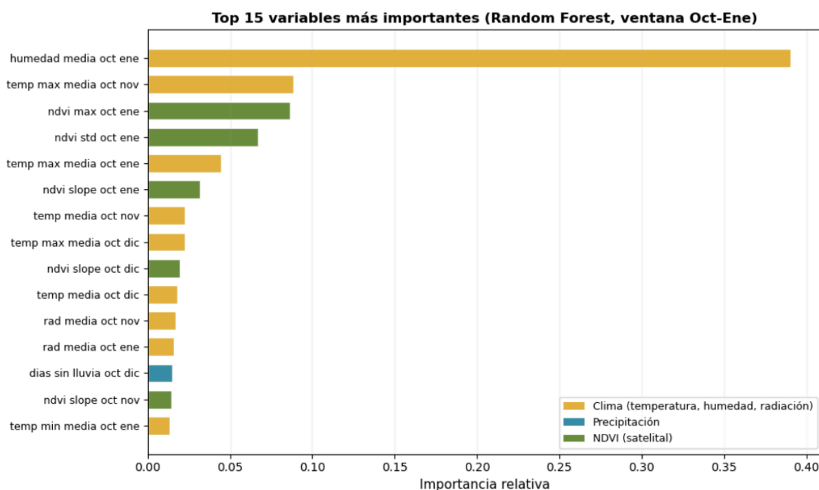
Figura 6. Top 15 variables con mayor importancia relativa en el modelo Random Forest (ventana octubre-enero). El color distingue el tipo de fuente: dorado para variables climáticas, verde para NDVI satelital y celeste para precipitación. Fuente: elaboración
