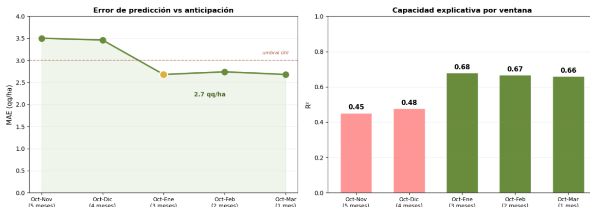
Figura 5. Error medio absoluto (izquierda) y coeficiente de determinación R^2 (derecha) del modelo Random Forest para cada ventana temporal. La línea punteada roja indica el umbral de error de 3 qq/ha considerado como referencia de utilidad. Fuente: elaboración propia.
