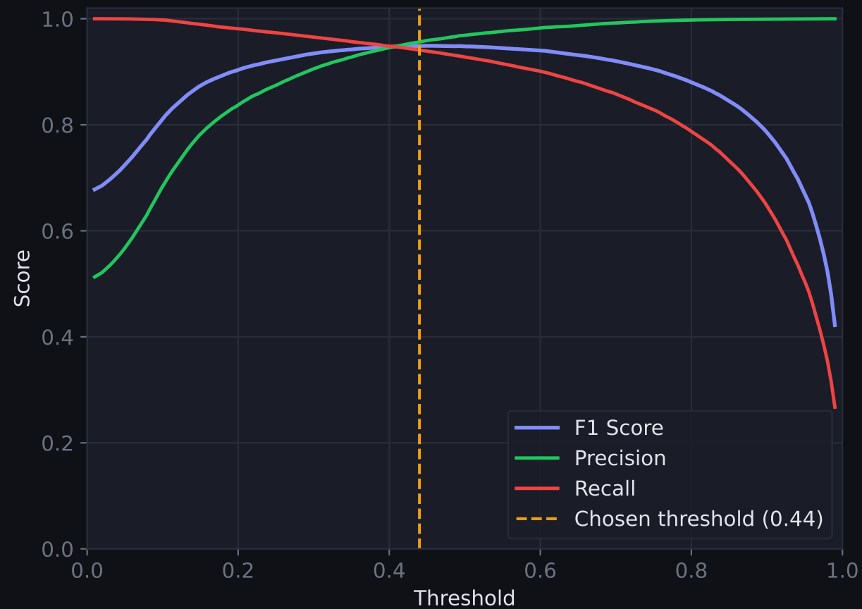
F1 / Precision / Recall vs Threshold
