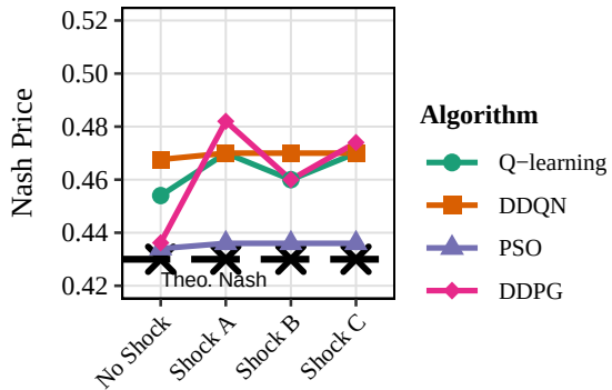
Linear
