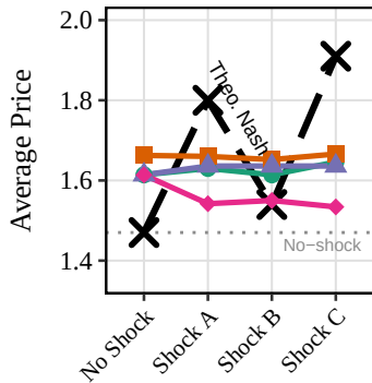
Logit
