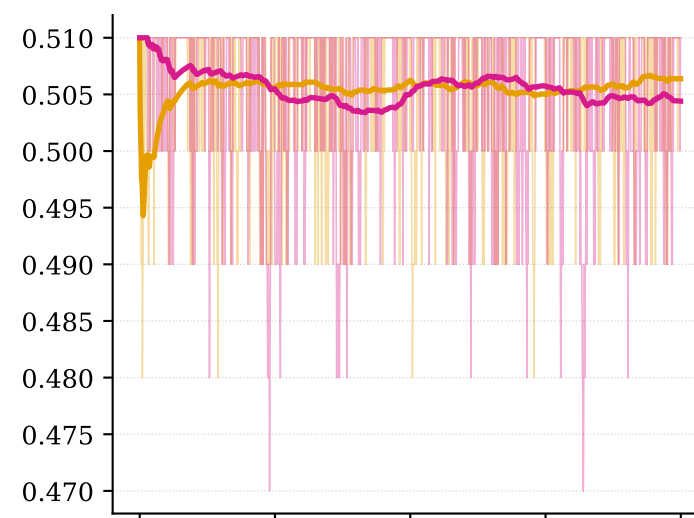
Linear
