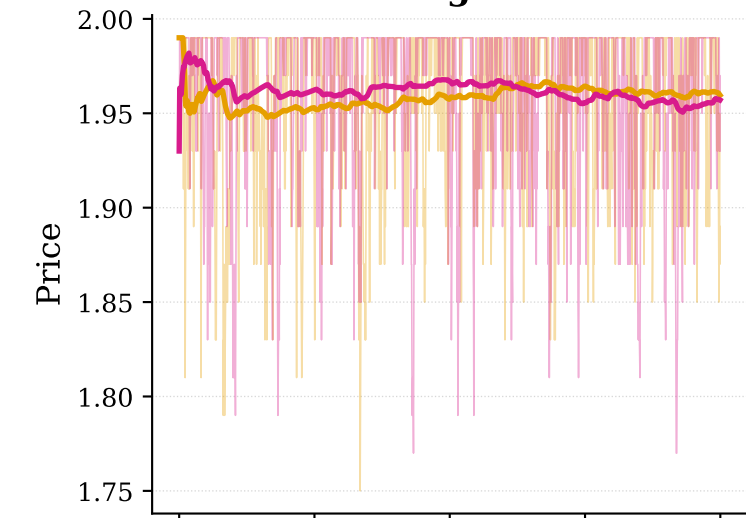
Logit
