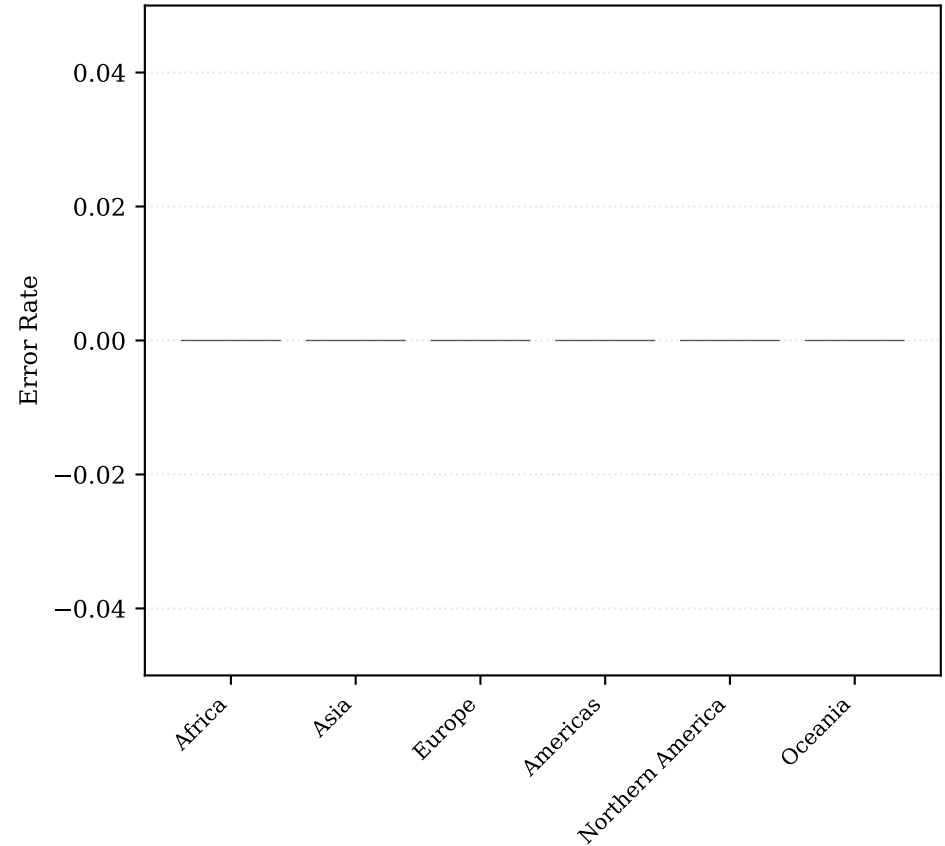
LLaVA-v1.6-7B
