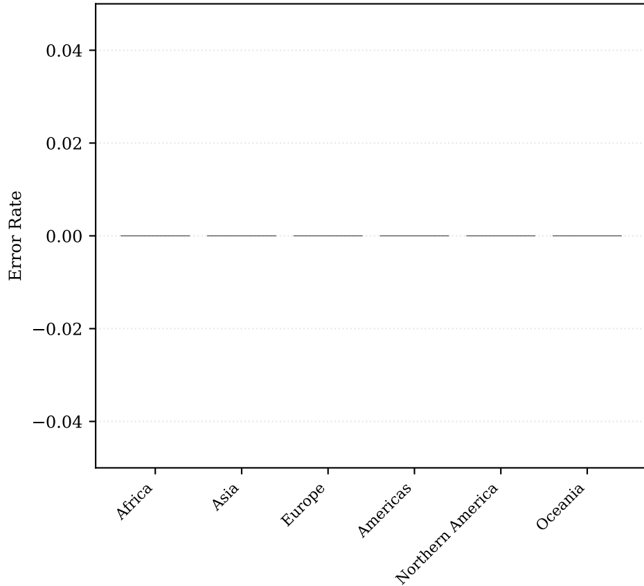
Llama-3.2-11B
